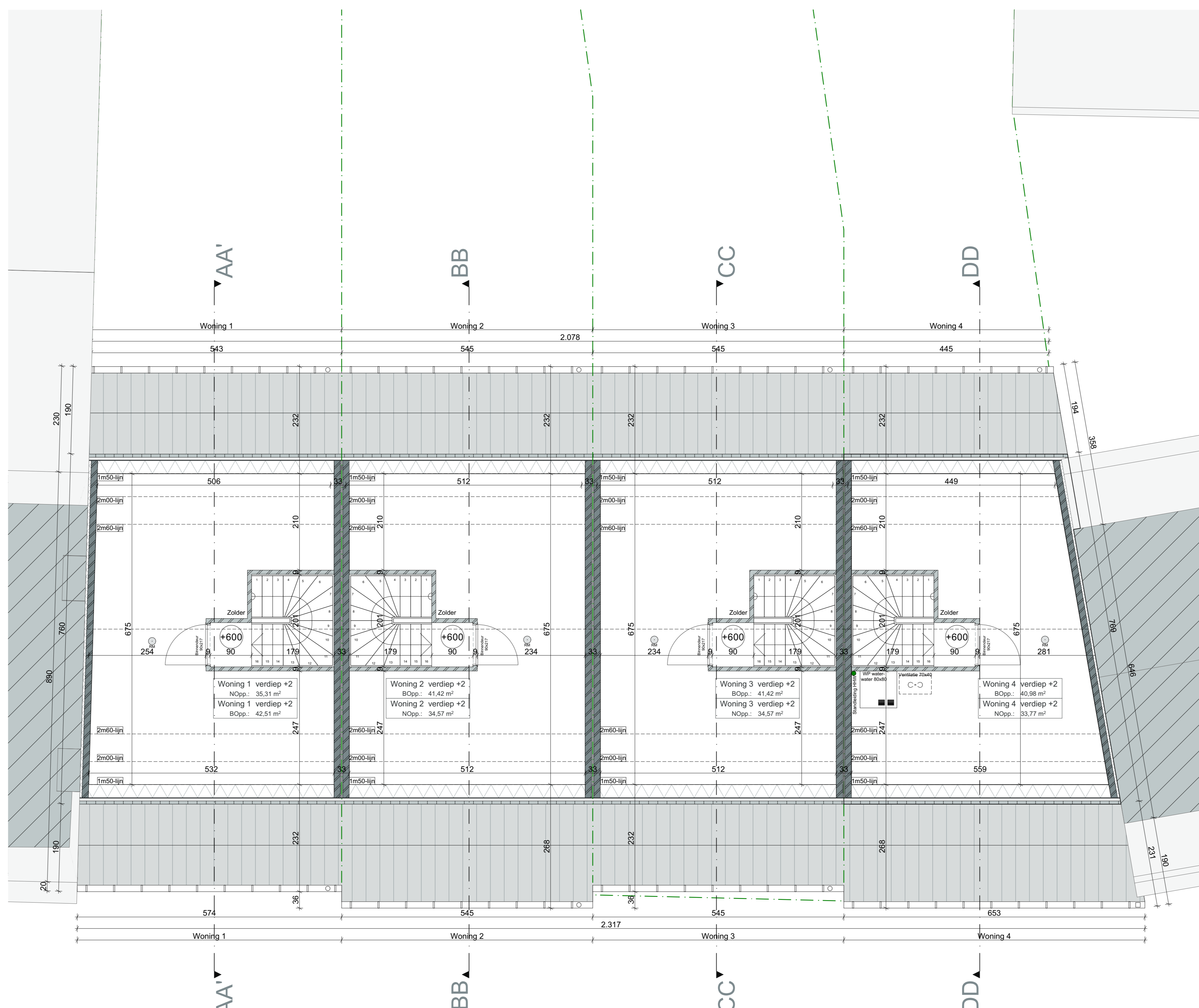
plan VERDIEP +2 1/50
