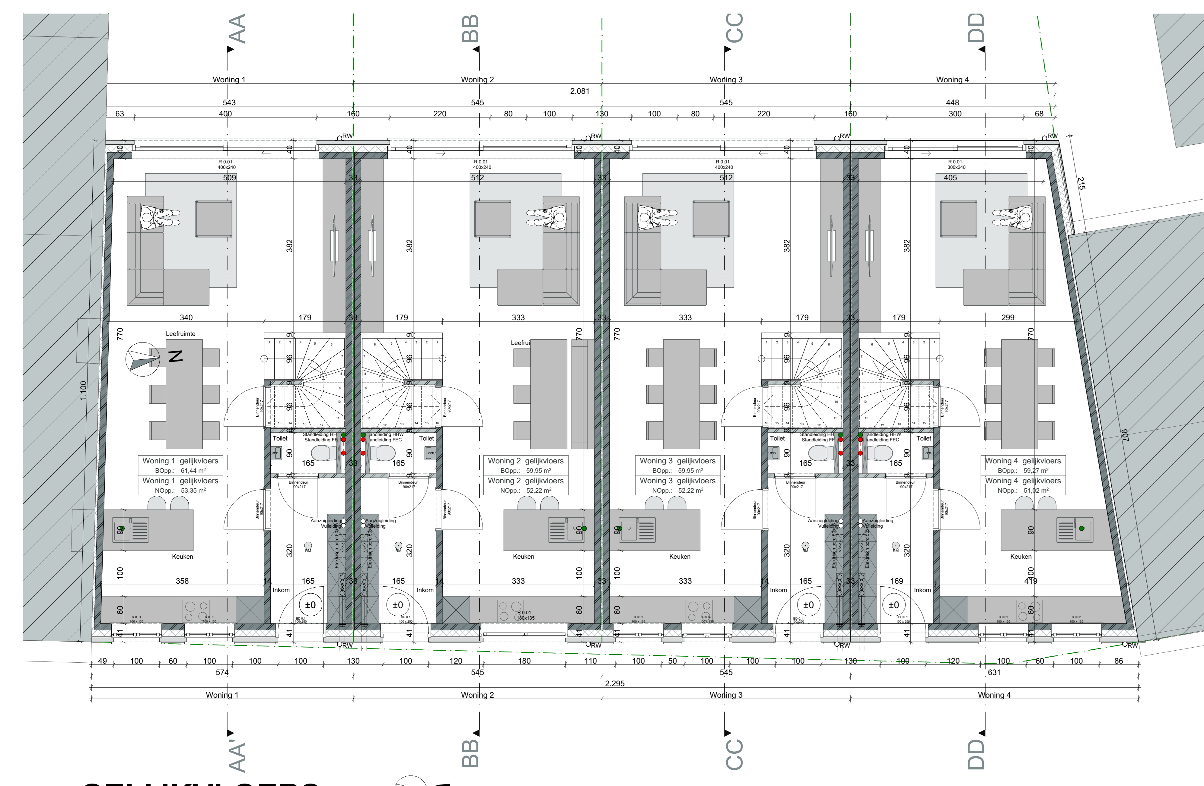
plan GELIJKVLOERS 1/50
