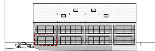
ELEVATION SUD-EST
