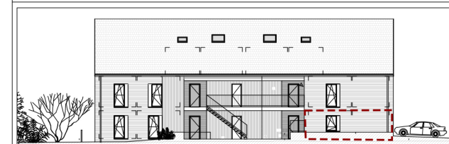
ELEVATION NORD-OUEST
