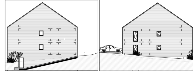
ELEVATION NORD-EST
