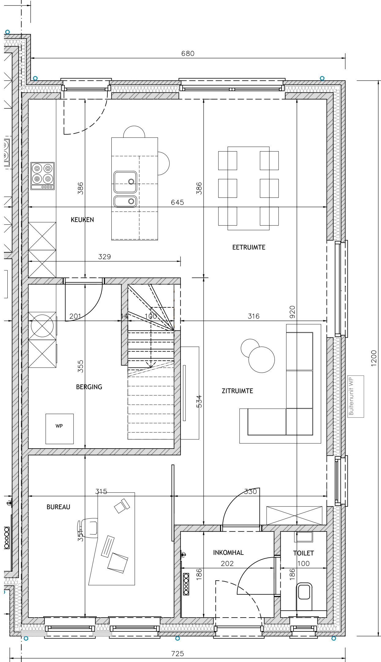
LOT 11 (Vogelzangstraat 2F) gelijkvloers schaal 1/50
