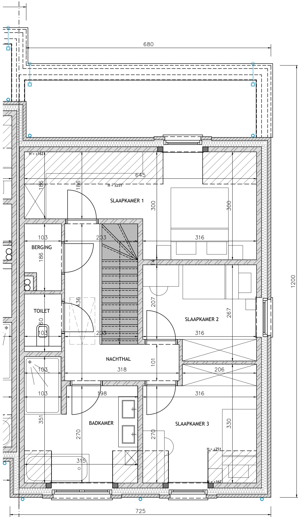
LOT 11 (Vogelzangstraat 2F) verdieping schaal 1/50
