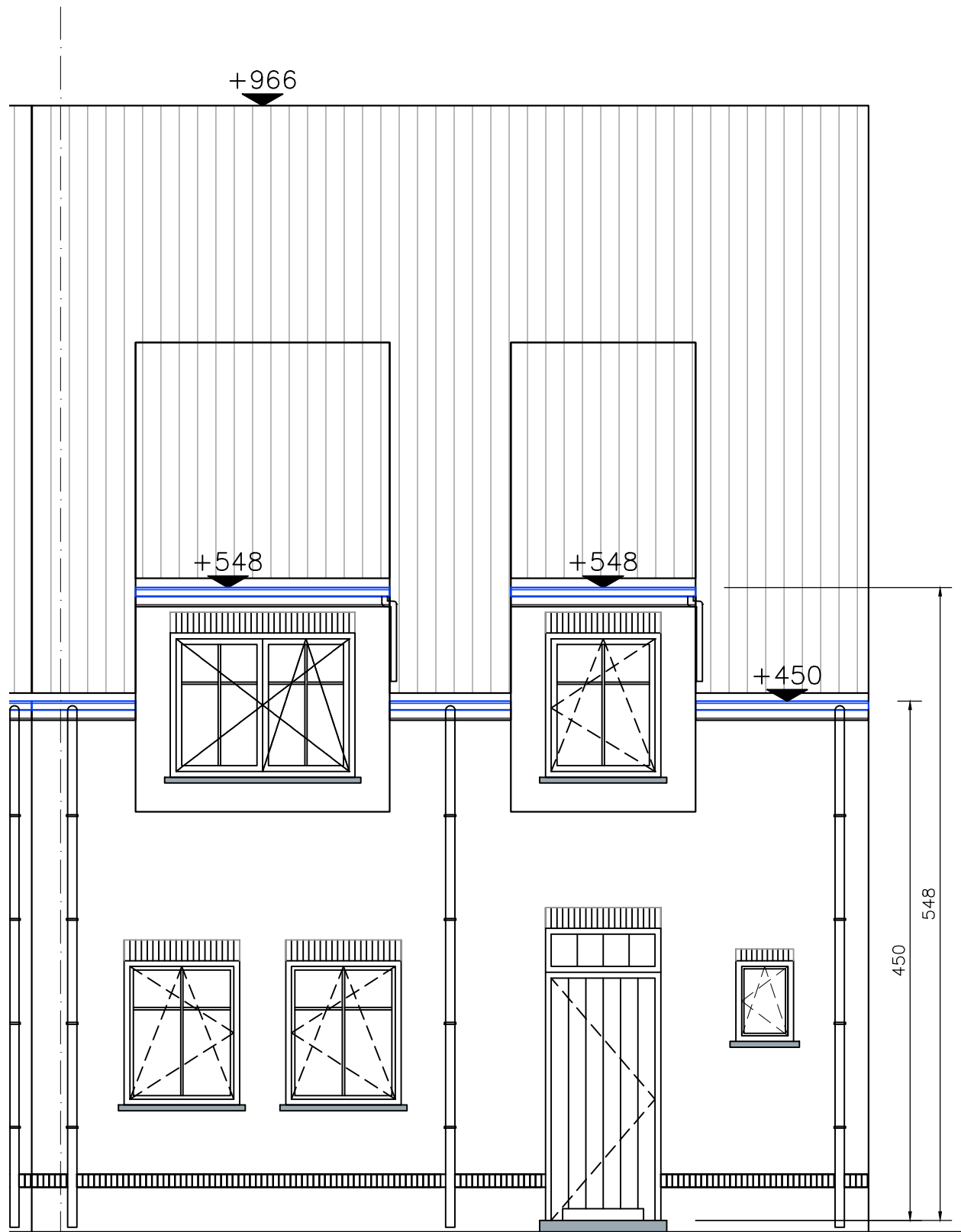
LOT 11 (Vogelzangstraat 2F) voorgevel schaal 1/50
