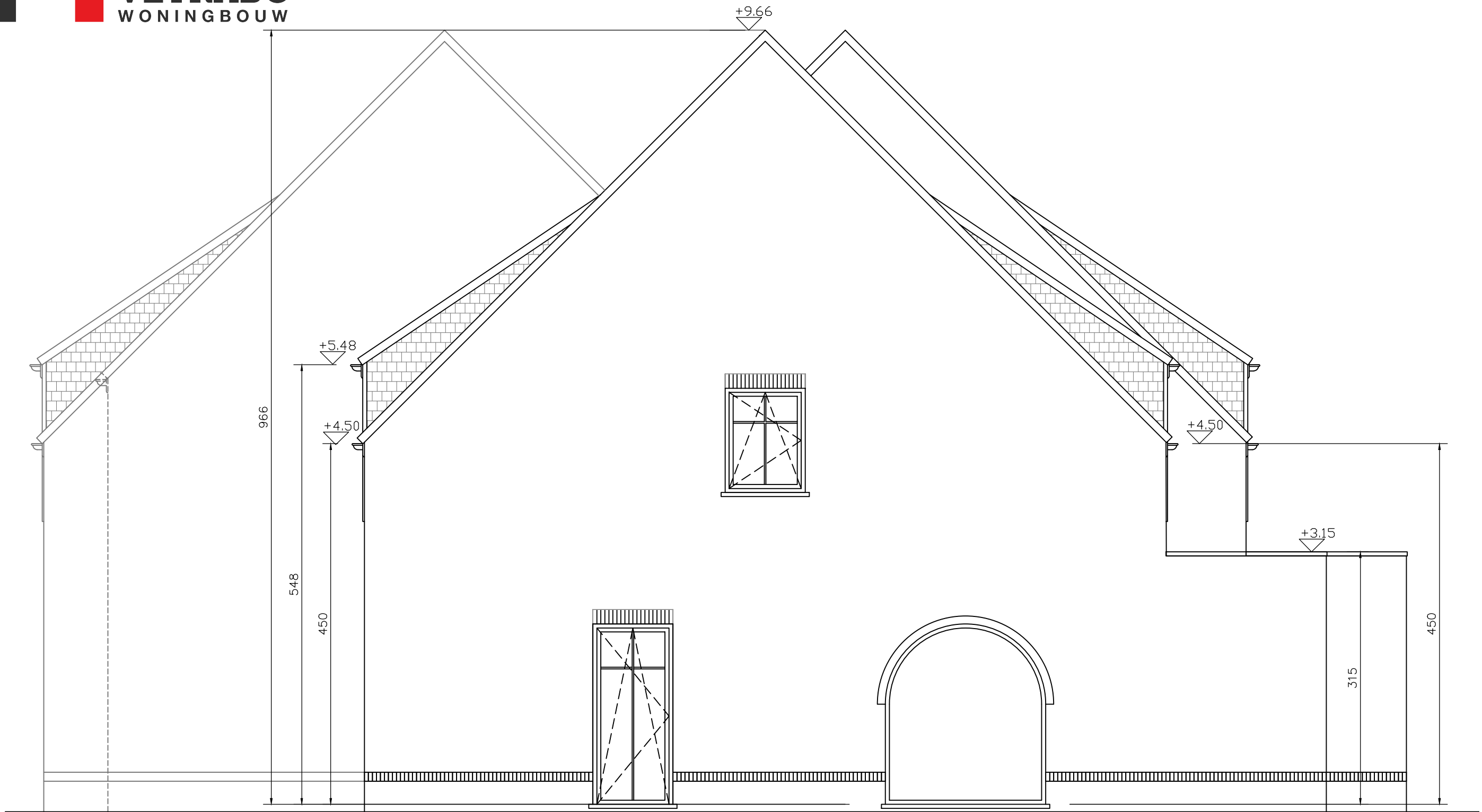
LOT 11 (Vogelzangstraat 2F) zijgevel rechts schaal 1/50
