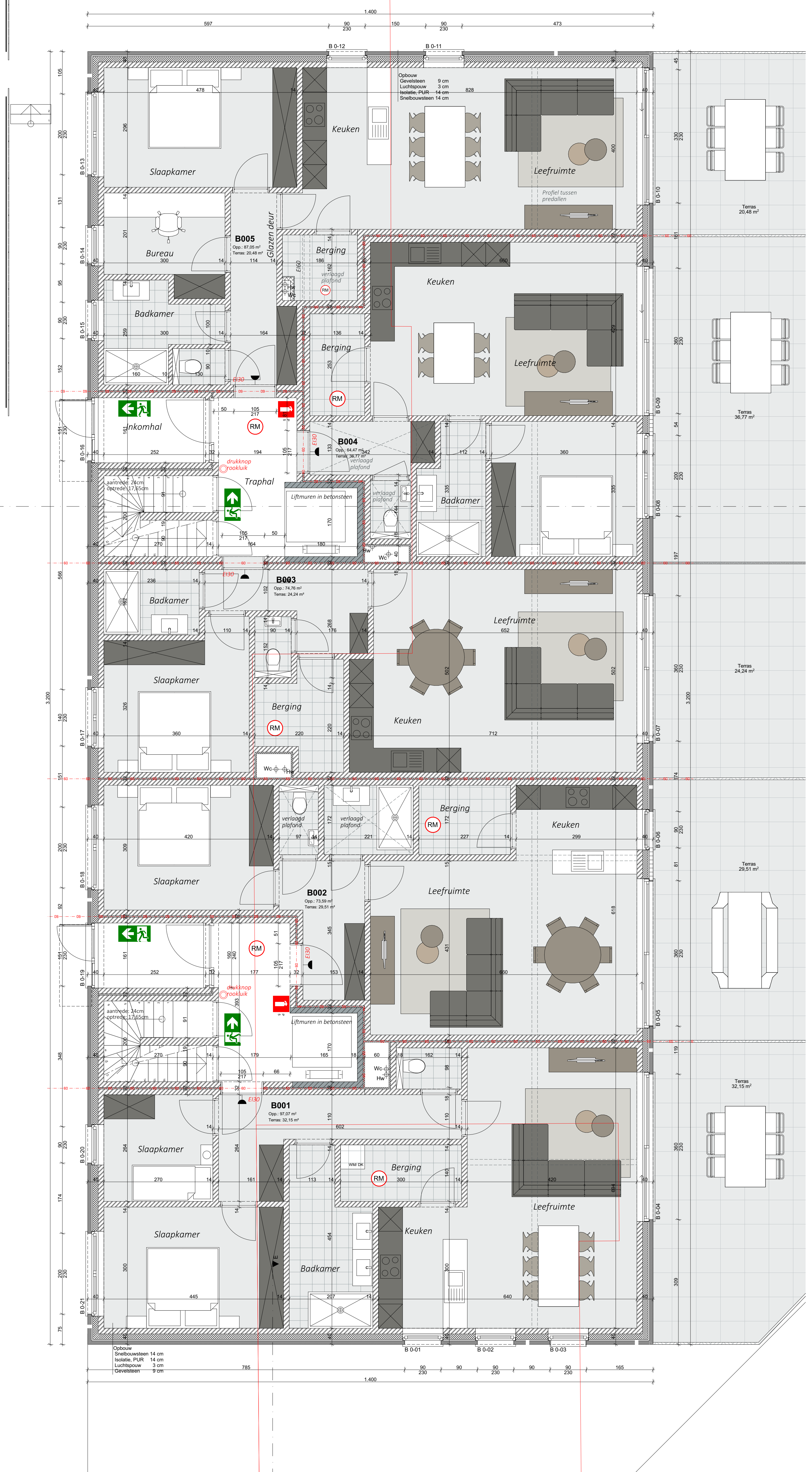
0B Gelijkvloers B
