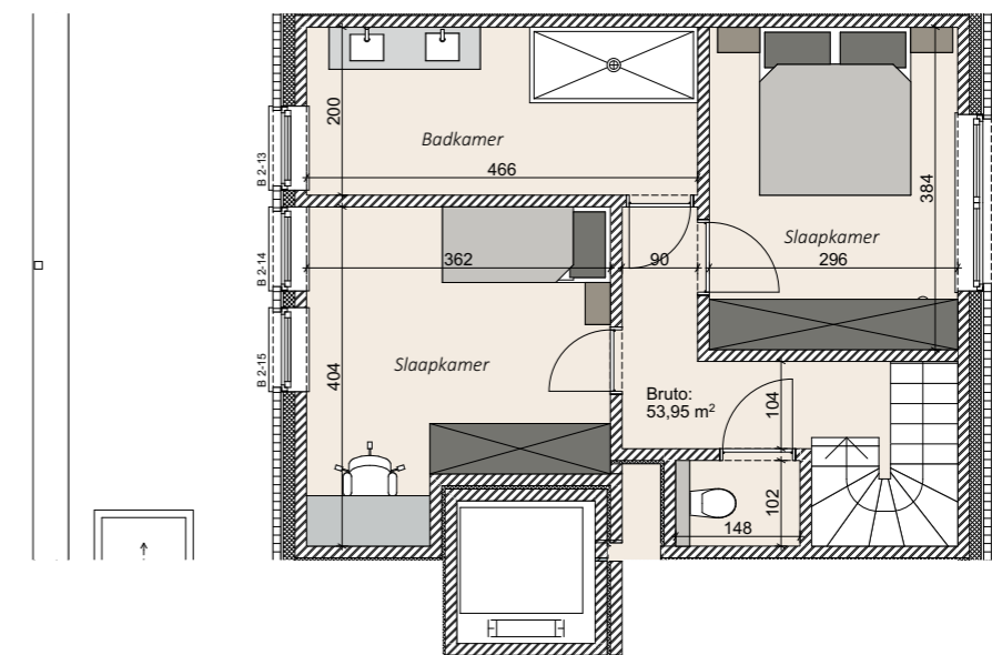
GRONDPLAN - 2e verdieping
