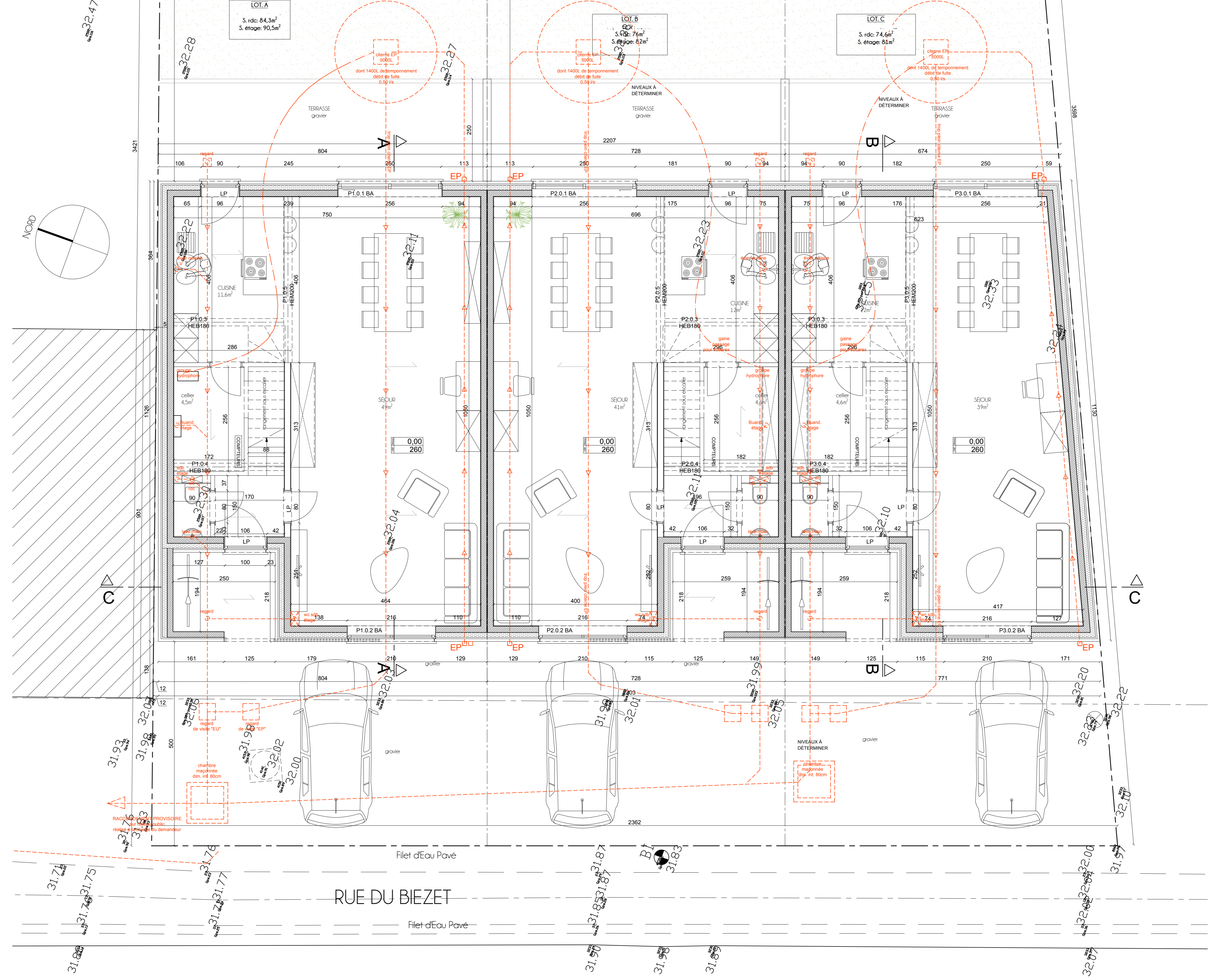
PLAN REZ-DE-CHAUSSEE éch. 1/50
