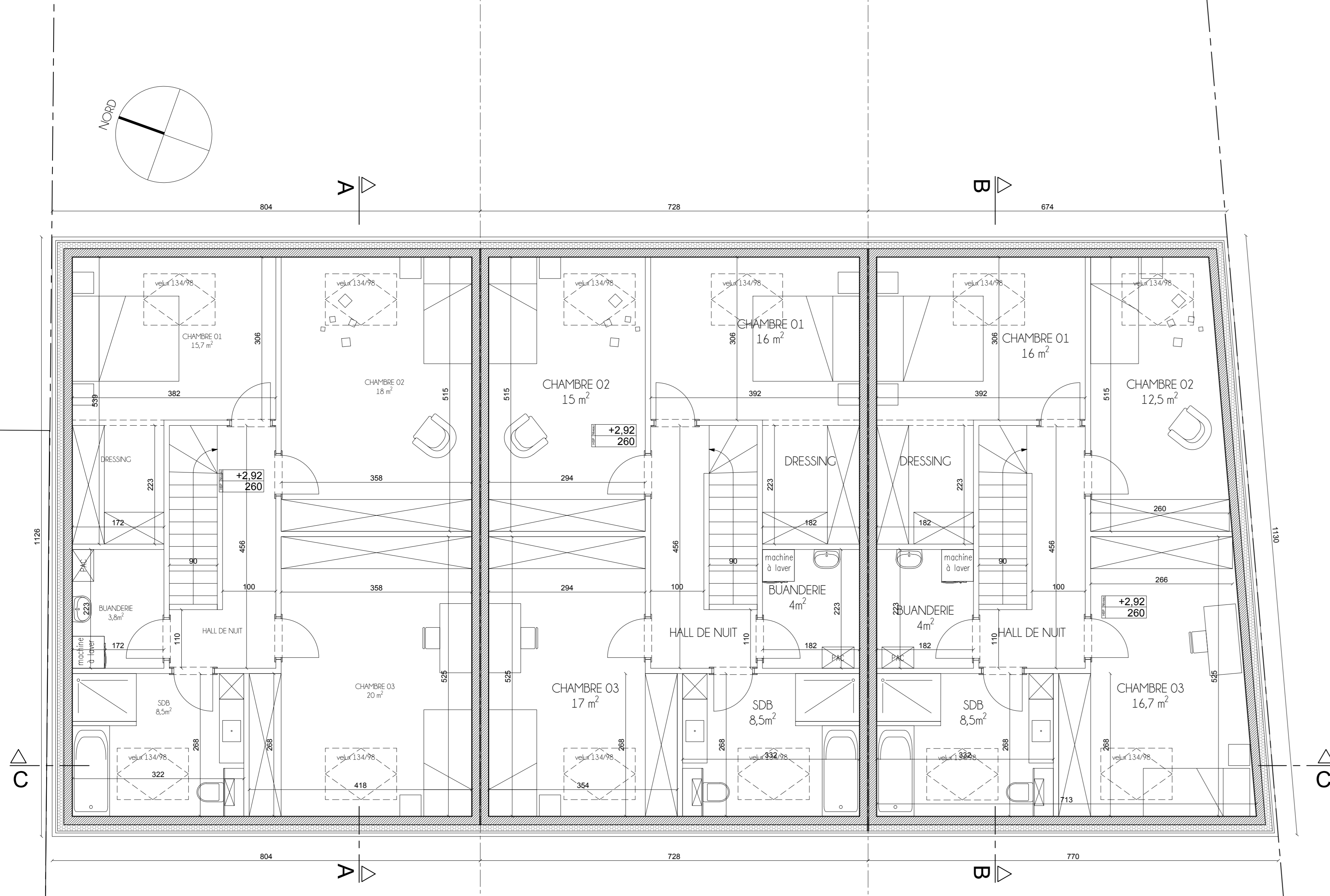
PLAN R+1 éch. 1/50
