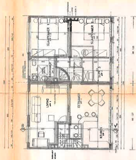
DERDE VERDIEPING
