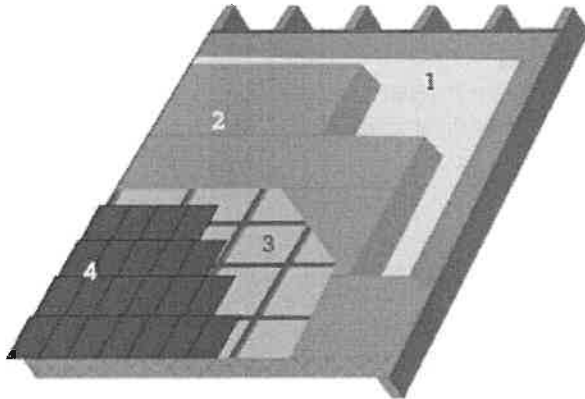
1. Damperschermbekleding | 2. Isolatie | 3. Onderdak | 4. Dakbedekking
