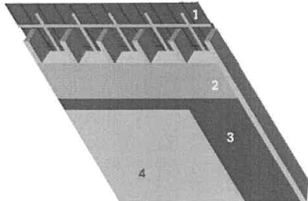
1. Onderdak | 2. Isolatie | 3. Damperschermbekleding | 4. binnenafwerking
