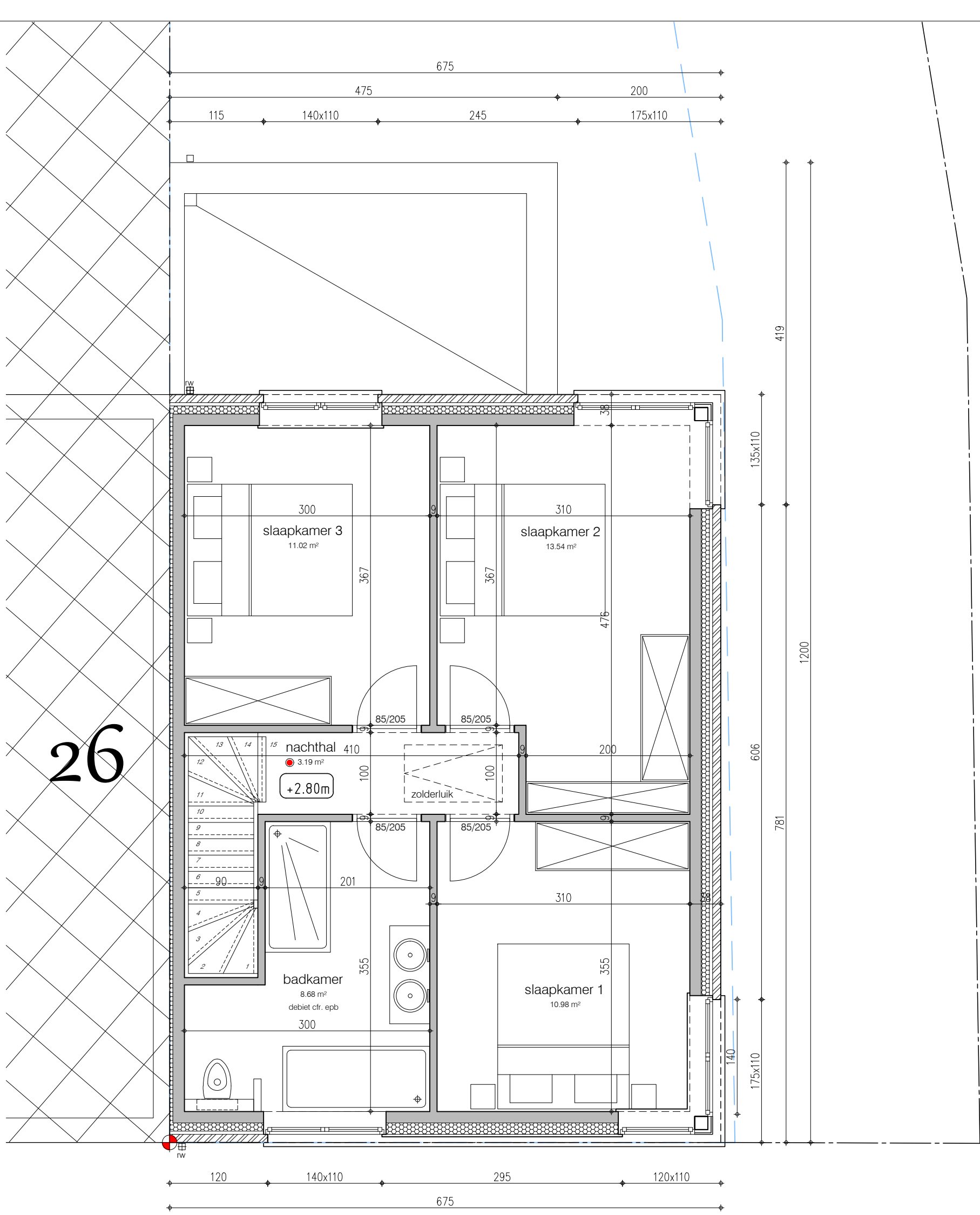
verdiepingsplan lot 1 61.83 m² brutto opp. 51.99 m² netto opp.
