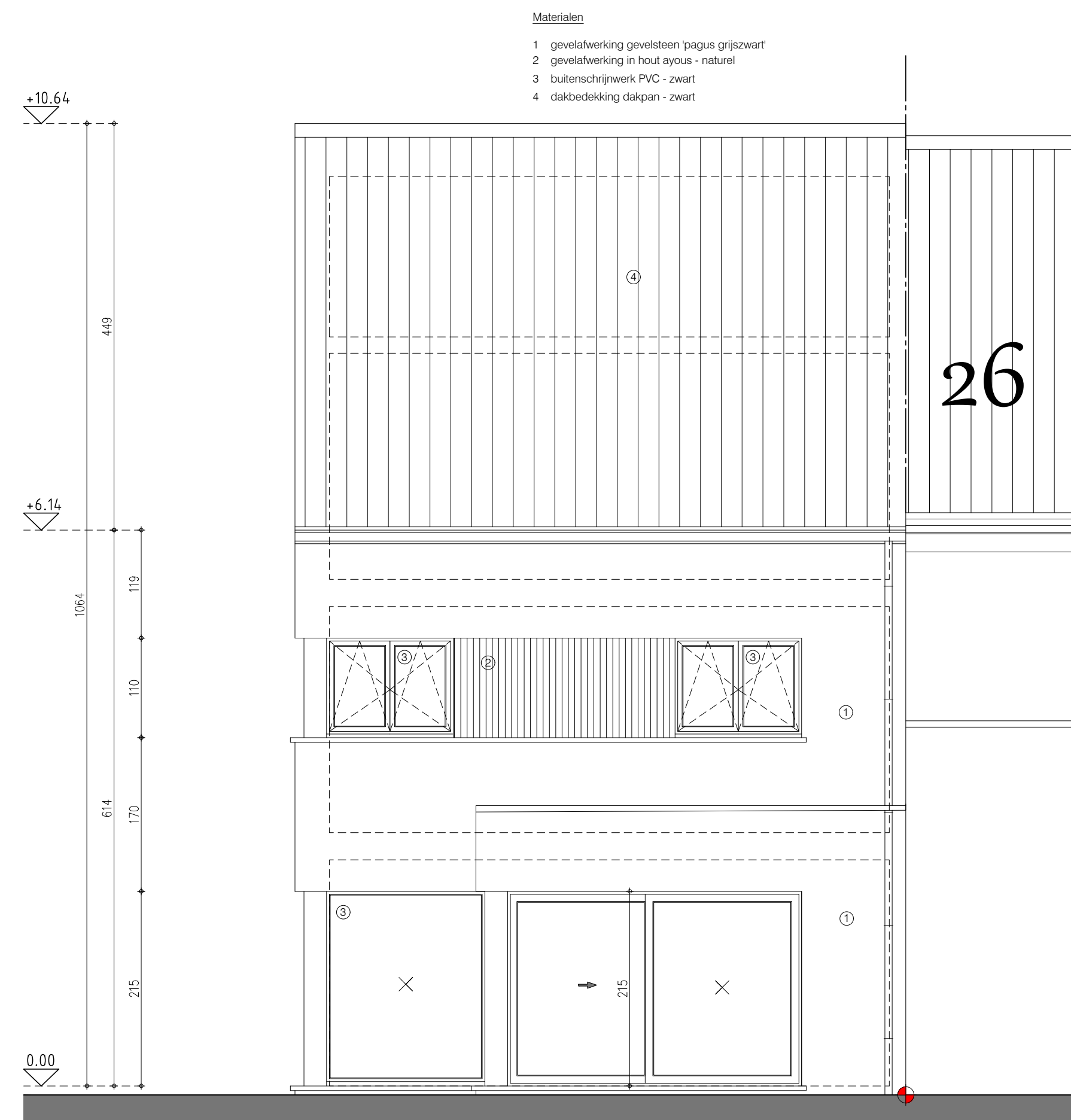
gevel zuid - achtergevel lot 1
