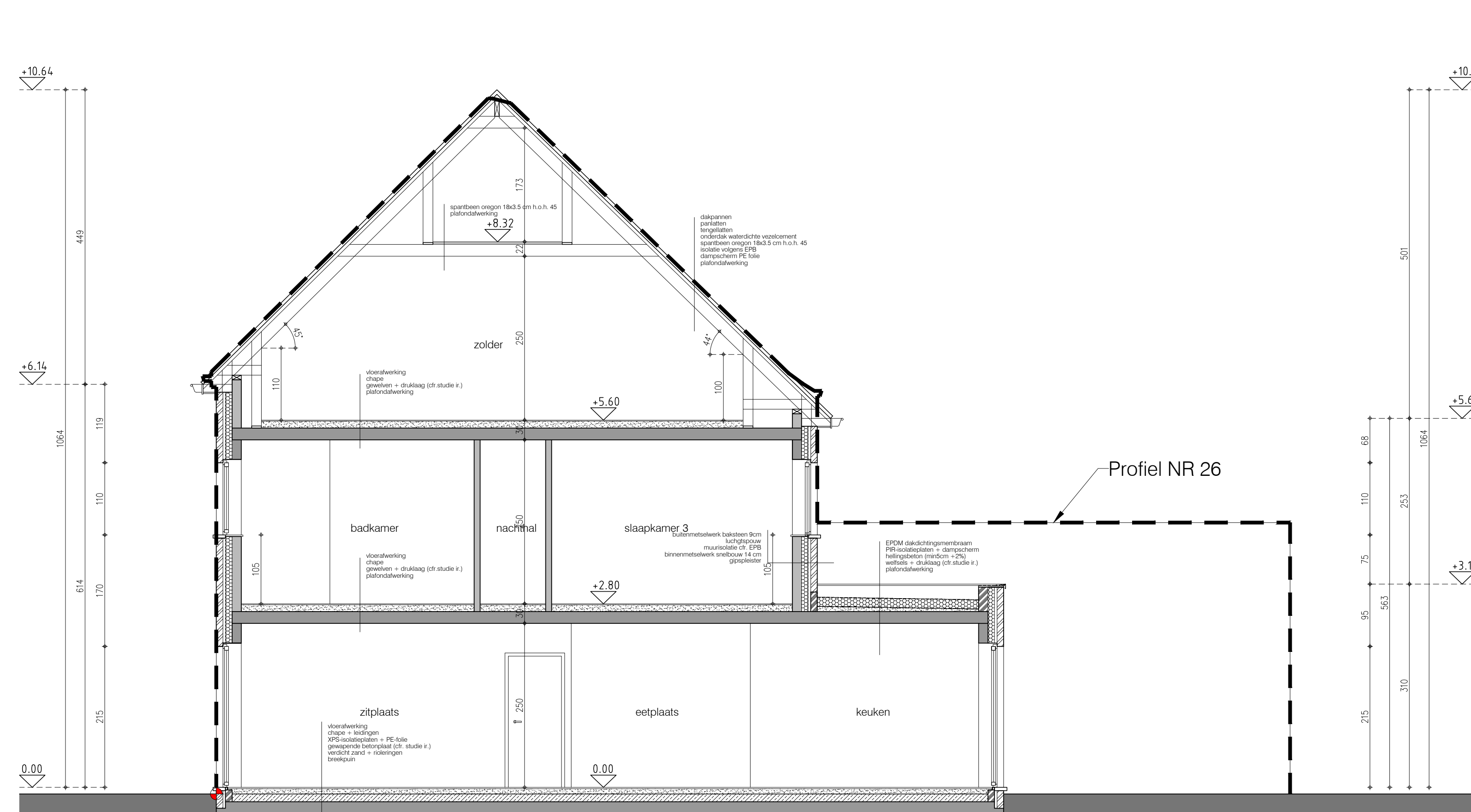
doorsnede 1-1
