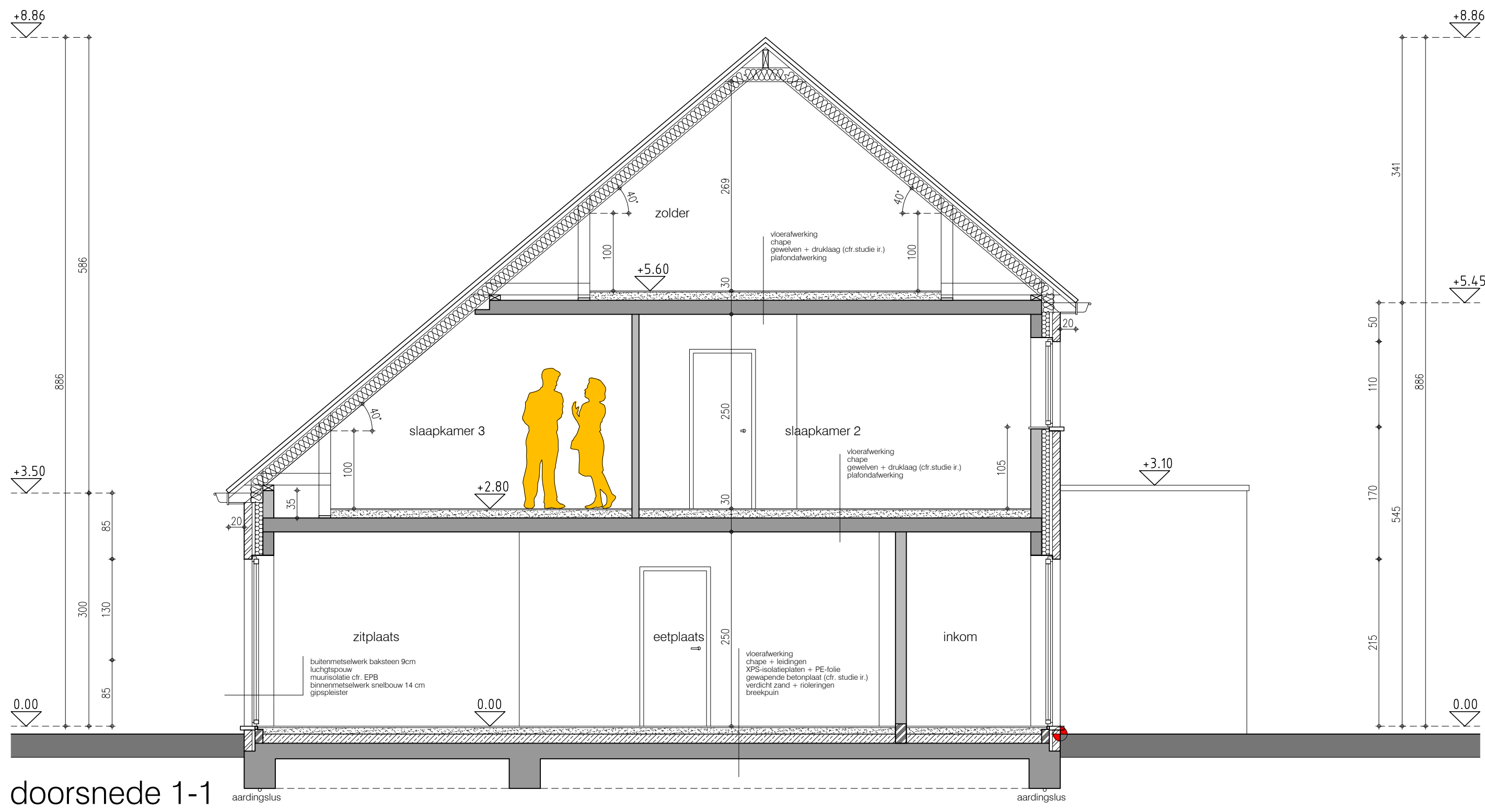
doorsnede 1-1
