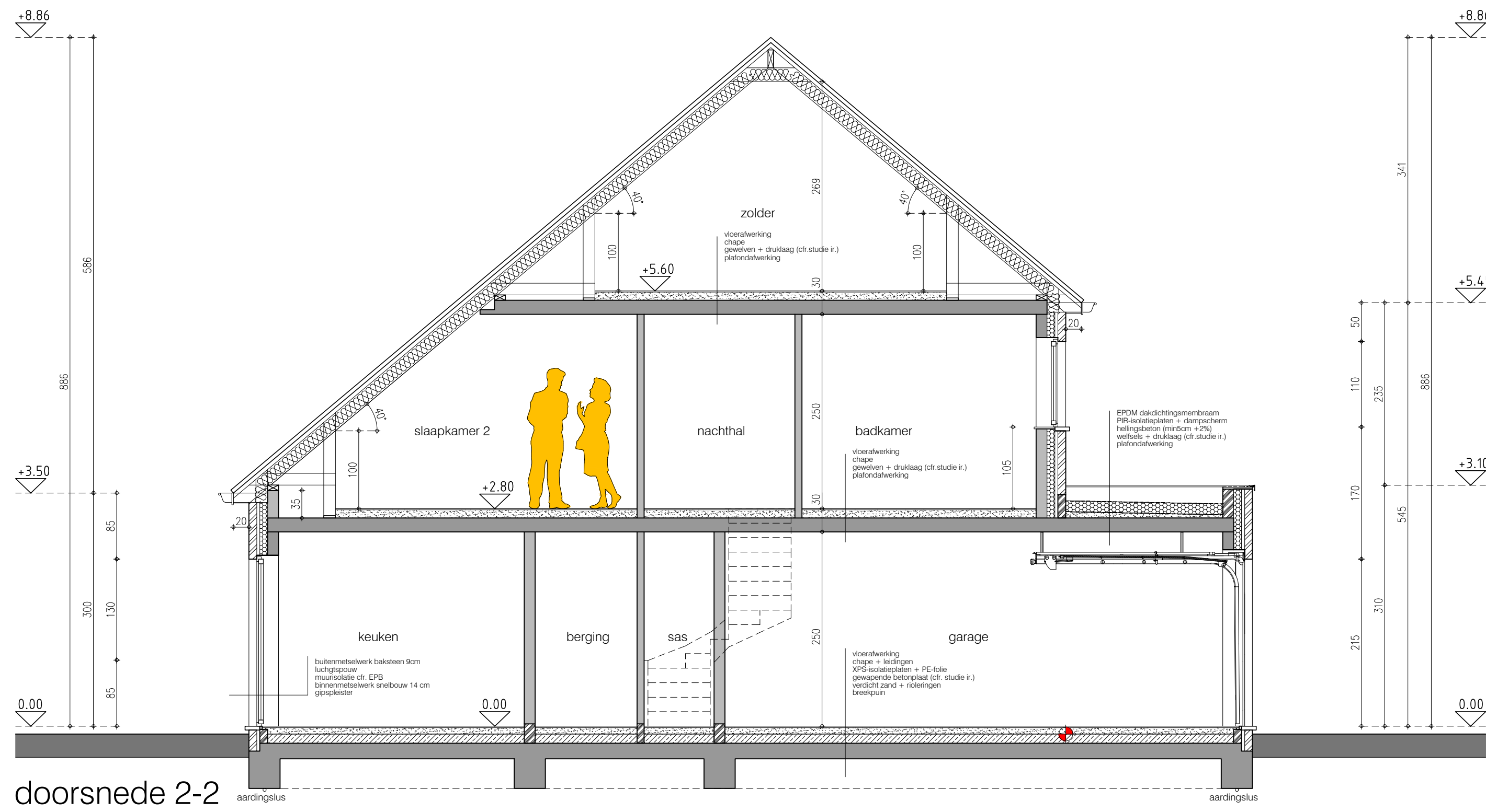
doorsnede 2-2
