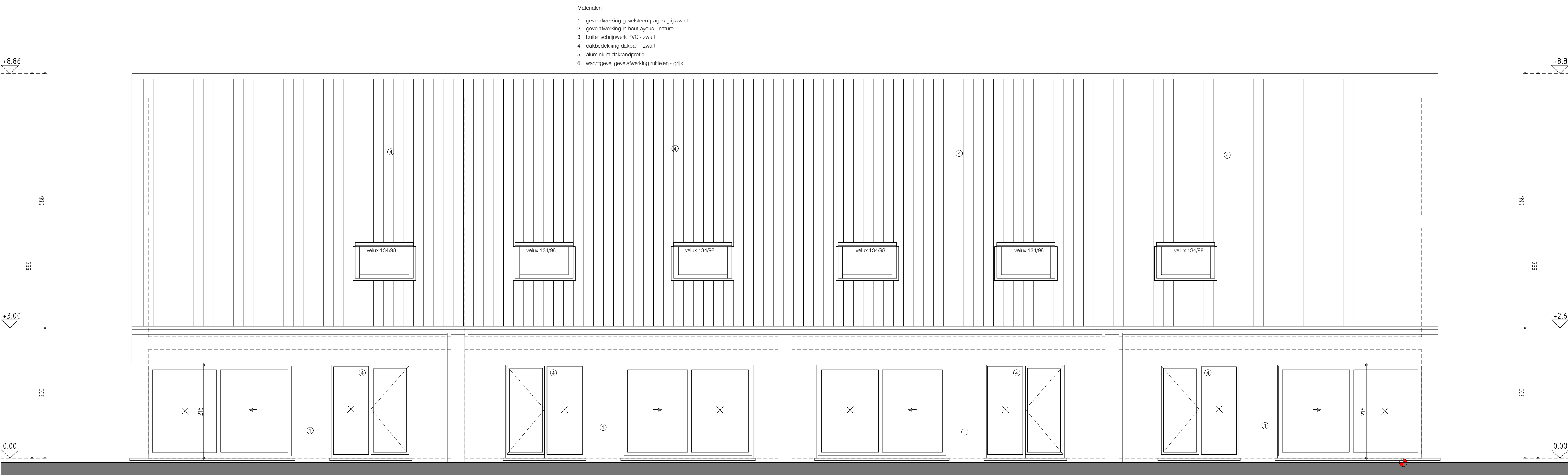
gevel west - achtergevel lot 14
