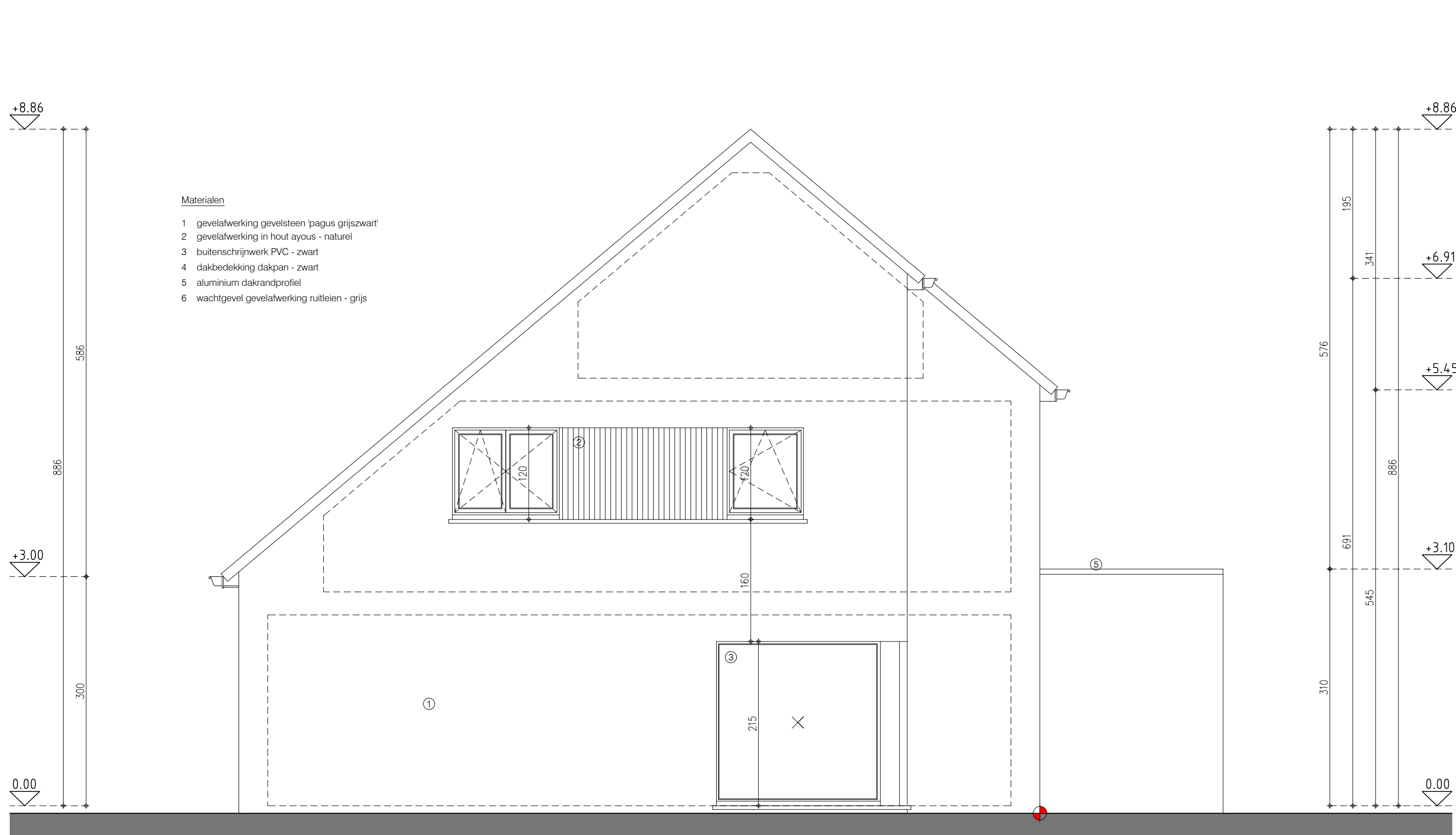
gevel zuid - linker zijgevel lot 11
