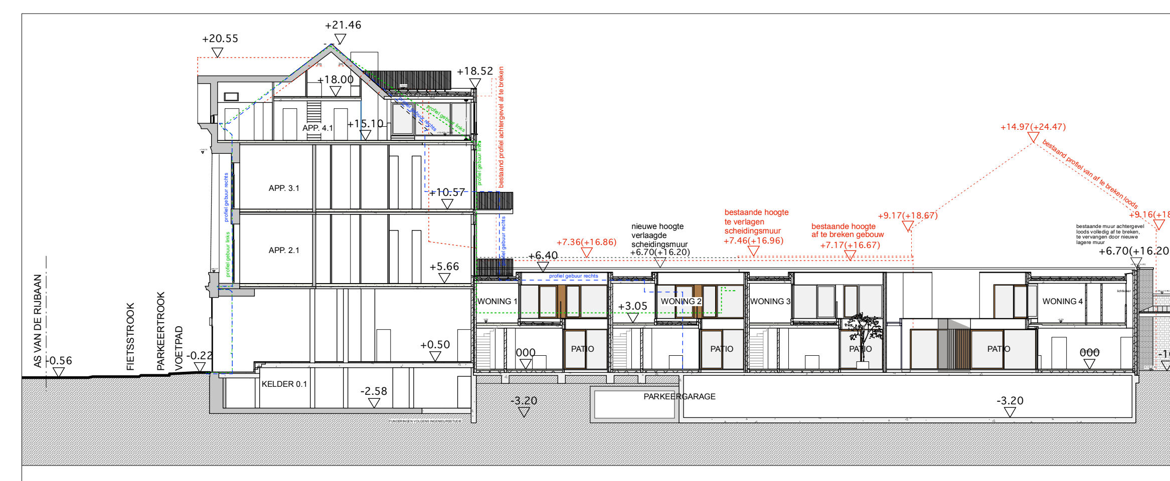
TERREINPROFIEL 1/250
