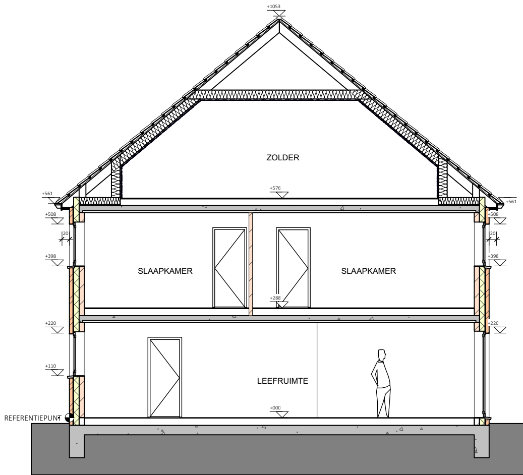
LANGSSNEDE 1/100
