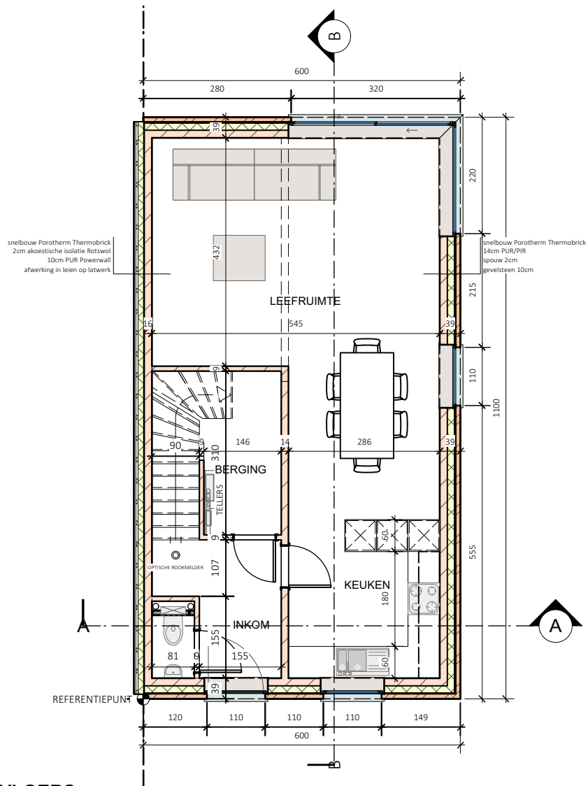
GELIJKVLOERS 1/100
