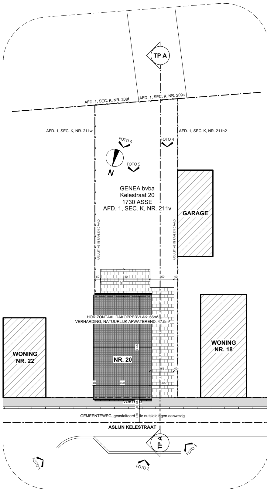
INPLANTINGSPLAN GEWENSTE TOESTAND 1/250
