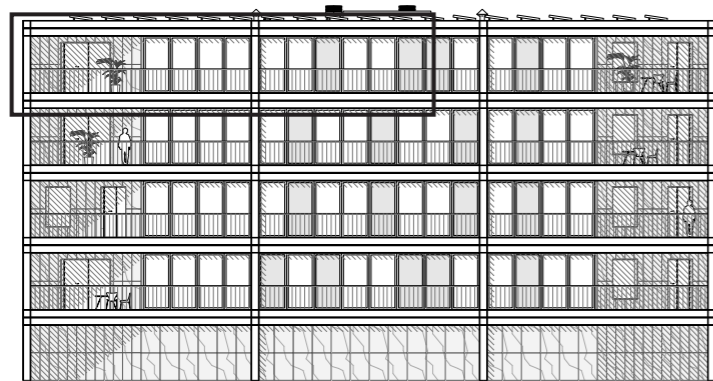
Noord gevel
