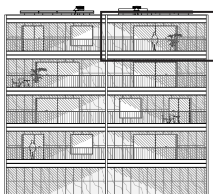
Oost gevel
