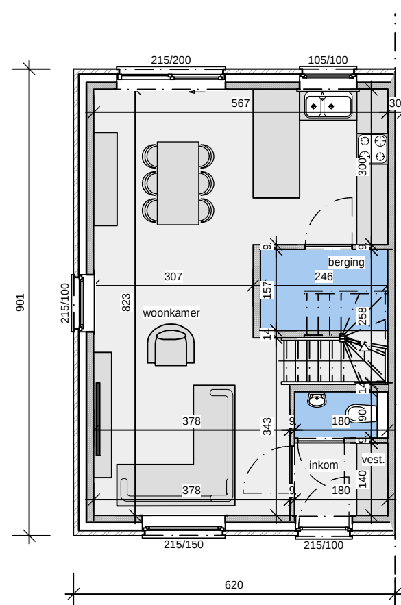
gelijkvloers 01 56m²
