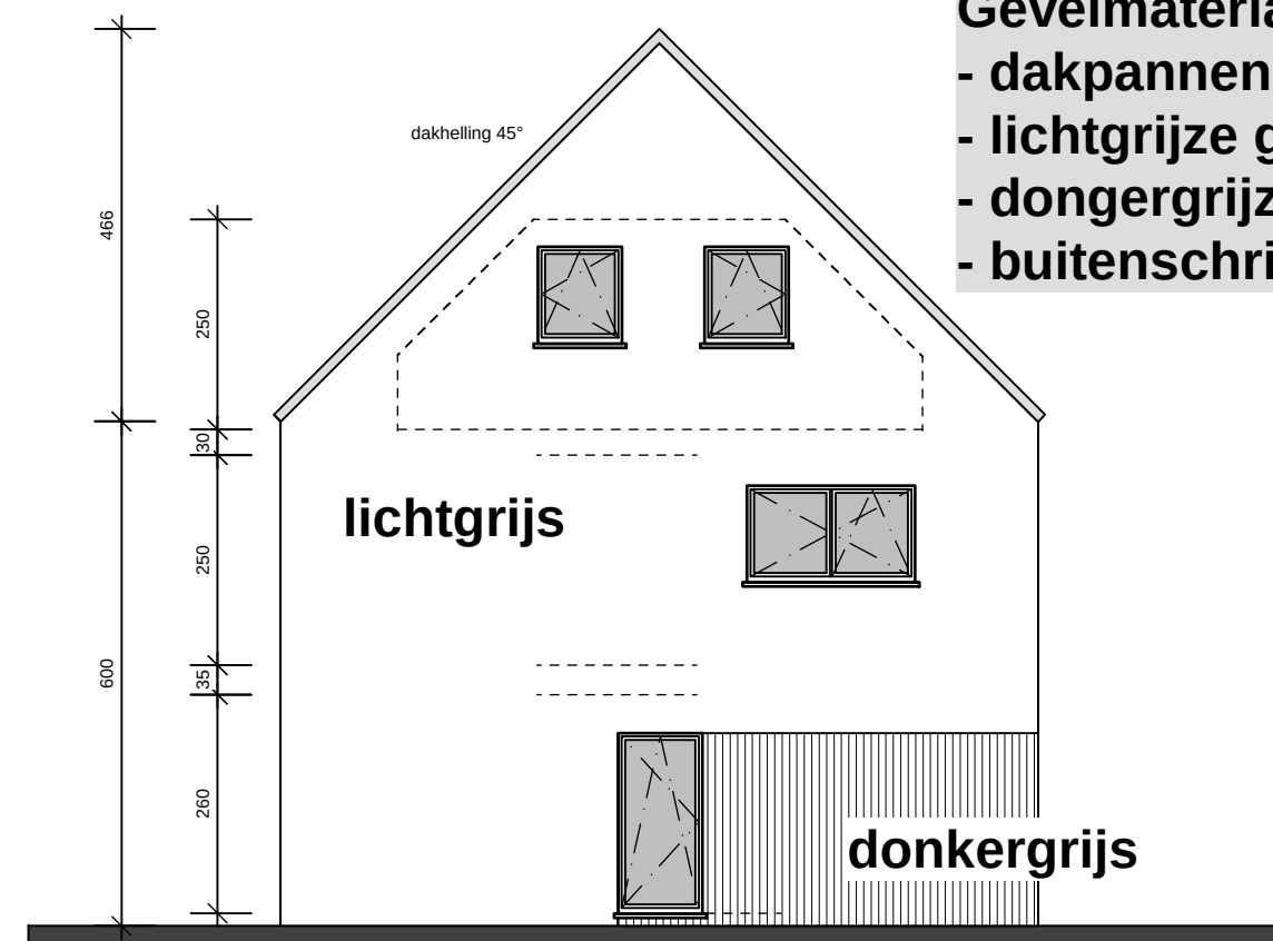
zijgevel links
