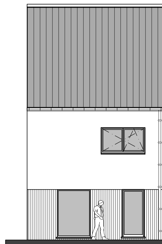
voorgevel
