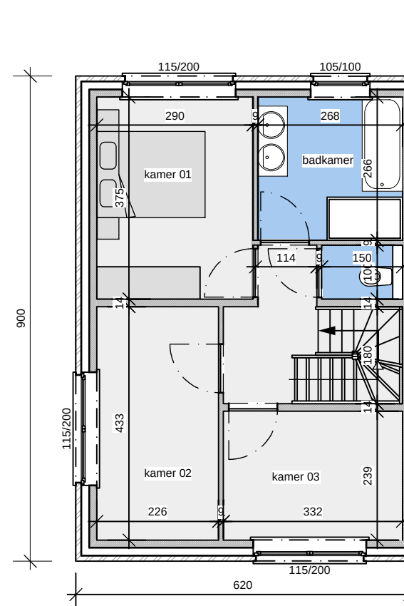
verdieping 01 56m²
