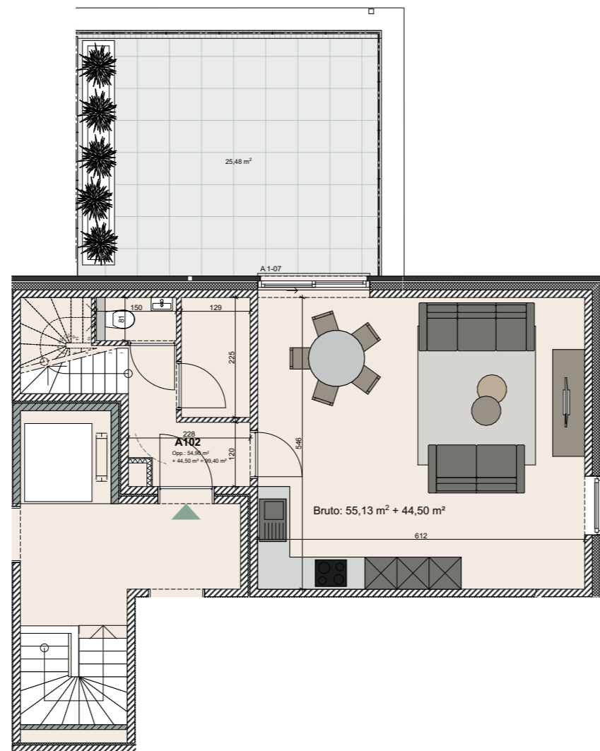
GRONDPLAN - 1 e verdieping
