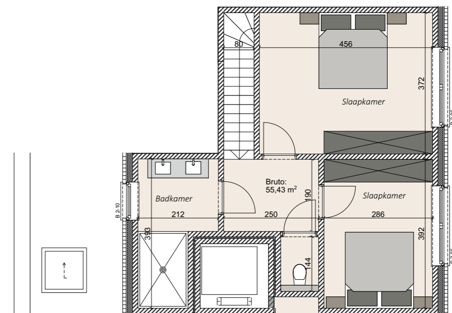
GRONDPLAN - 2e verdieping
