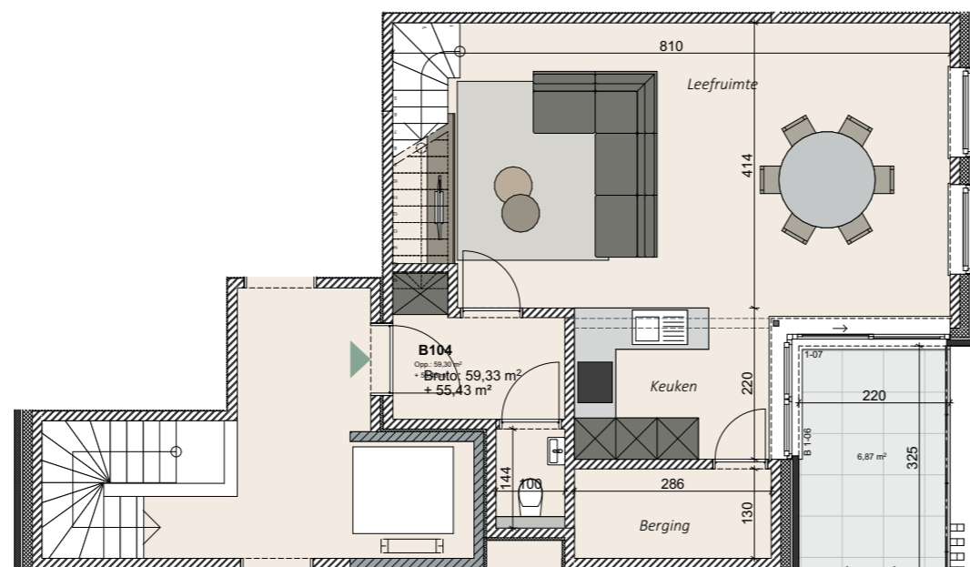
GRONDPLAN - 1e verdieping
