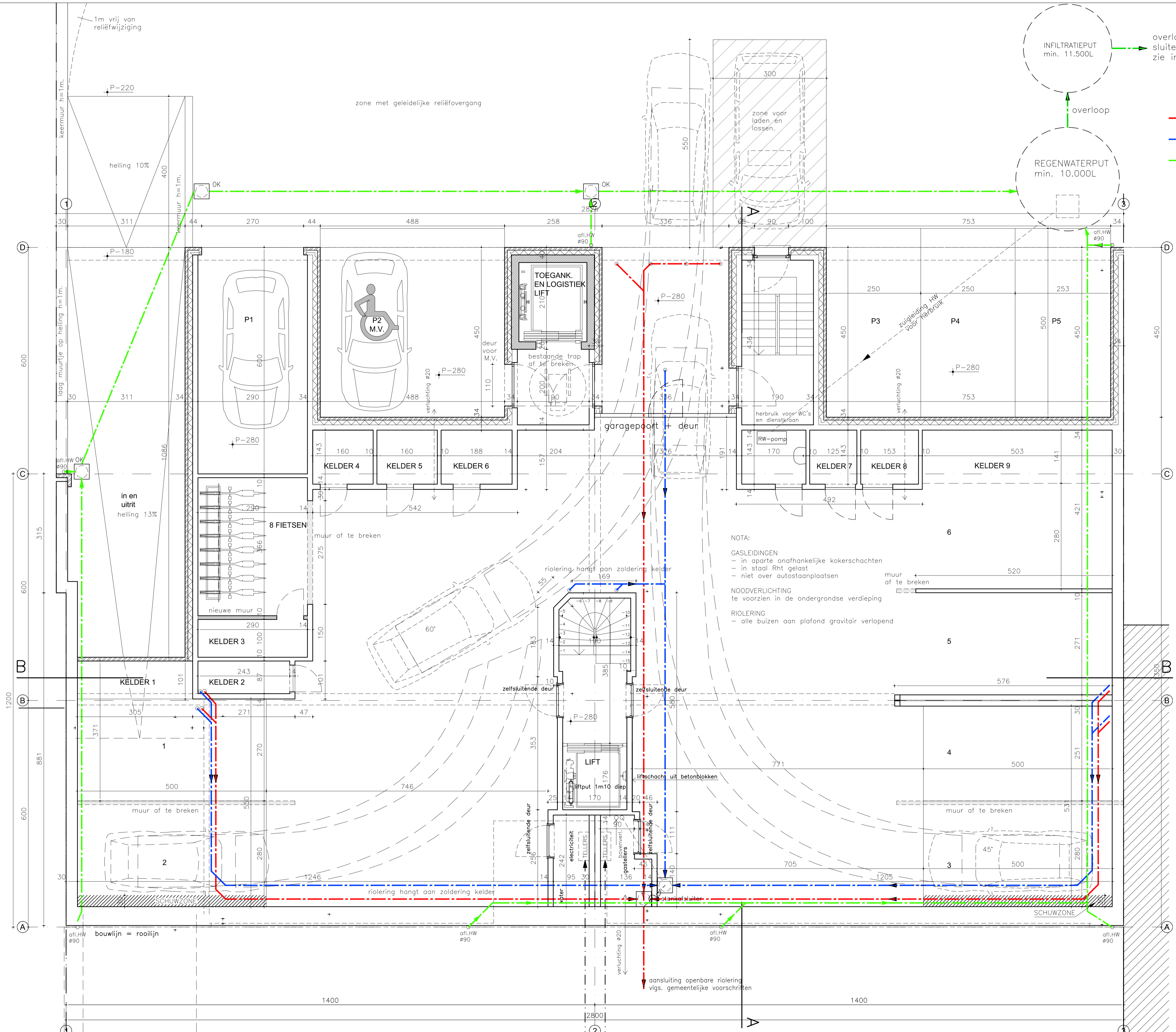
KELDER + RIOLERING - VERGUNDE TOESTAND
