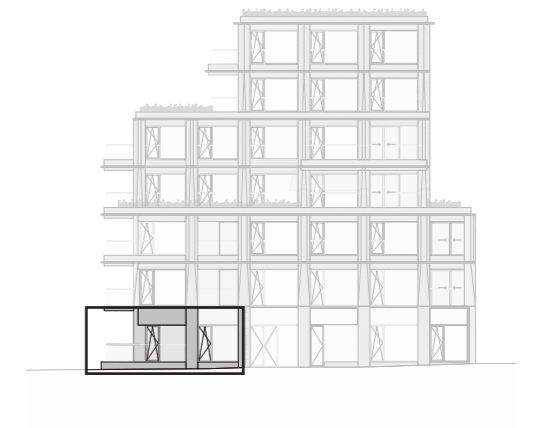
Oostgevel 1/500
