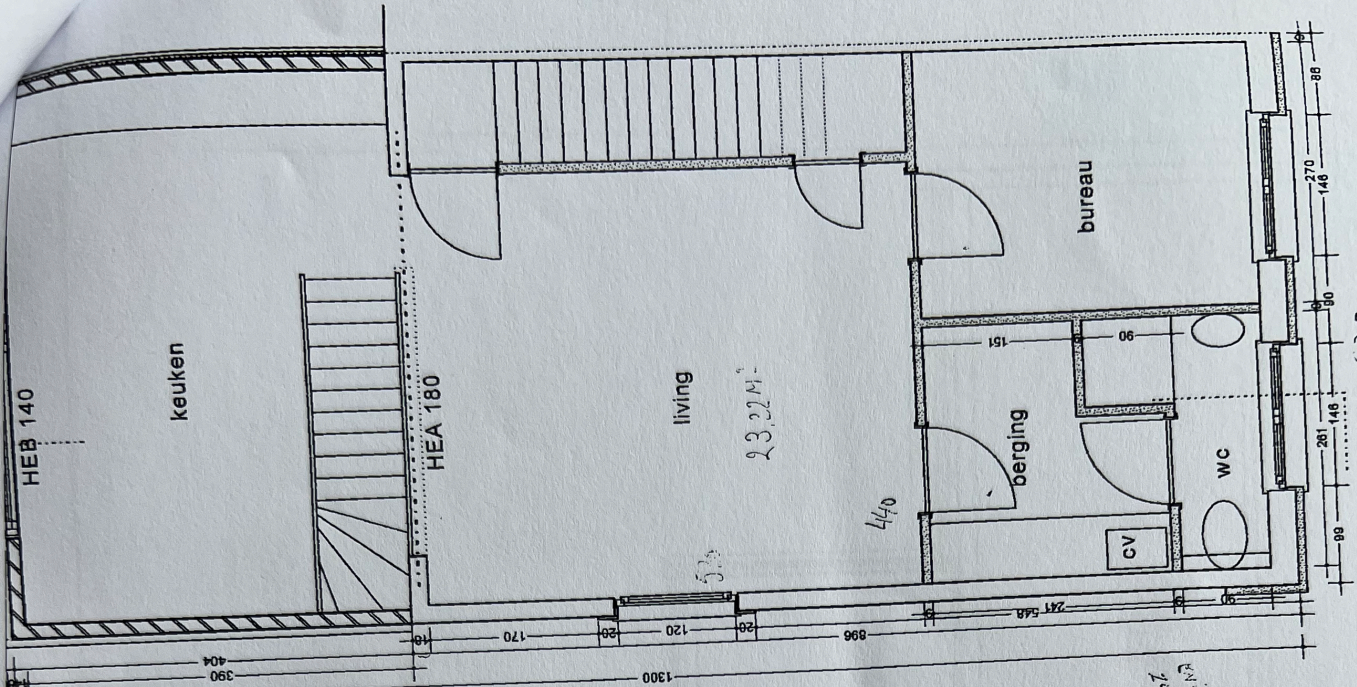
GRONDPLAN VERDIEPING 1
