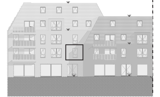
Noordwestengevel 1/500
