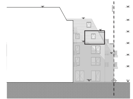
Noordoostengevel 1/500
