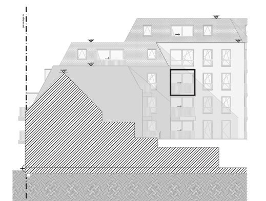
Zuidwestengevel 1/500
