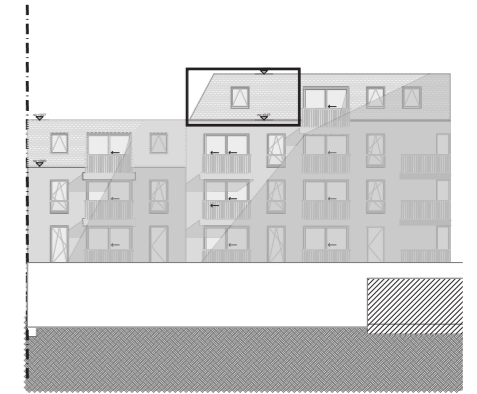
Zuidoostengevel 1/500
