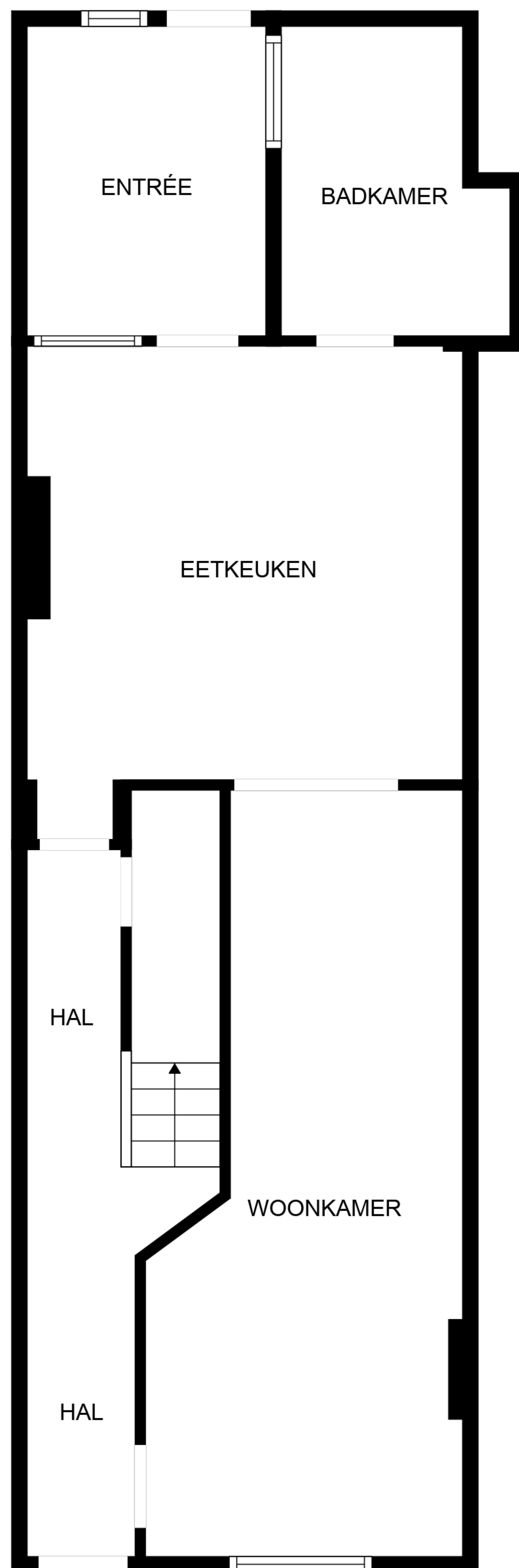
1. VERDIEPING
