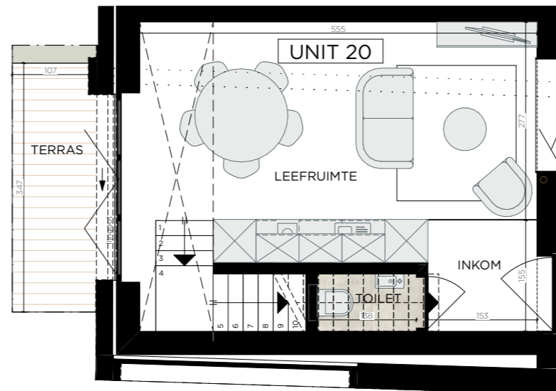
GELIJKVLOERS
