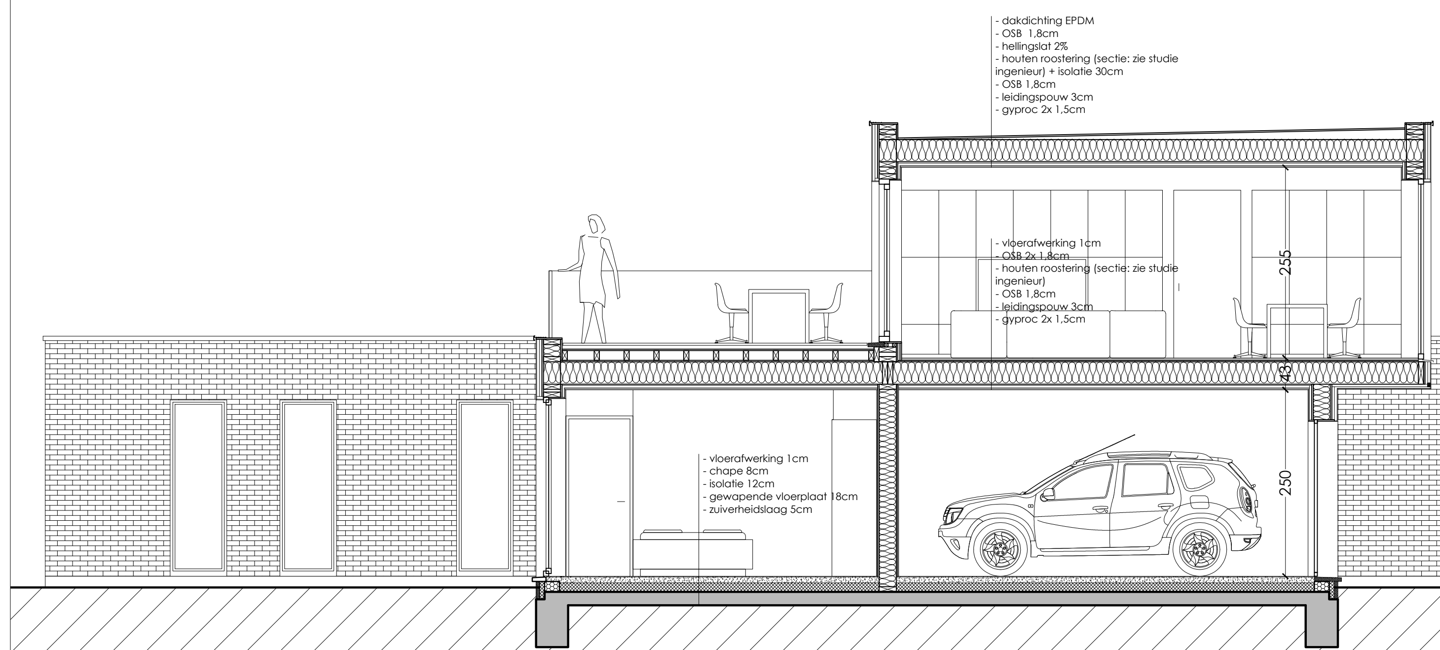
DOORSNEDE AA' _ 1/50
