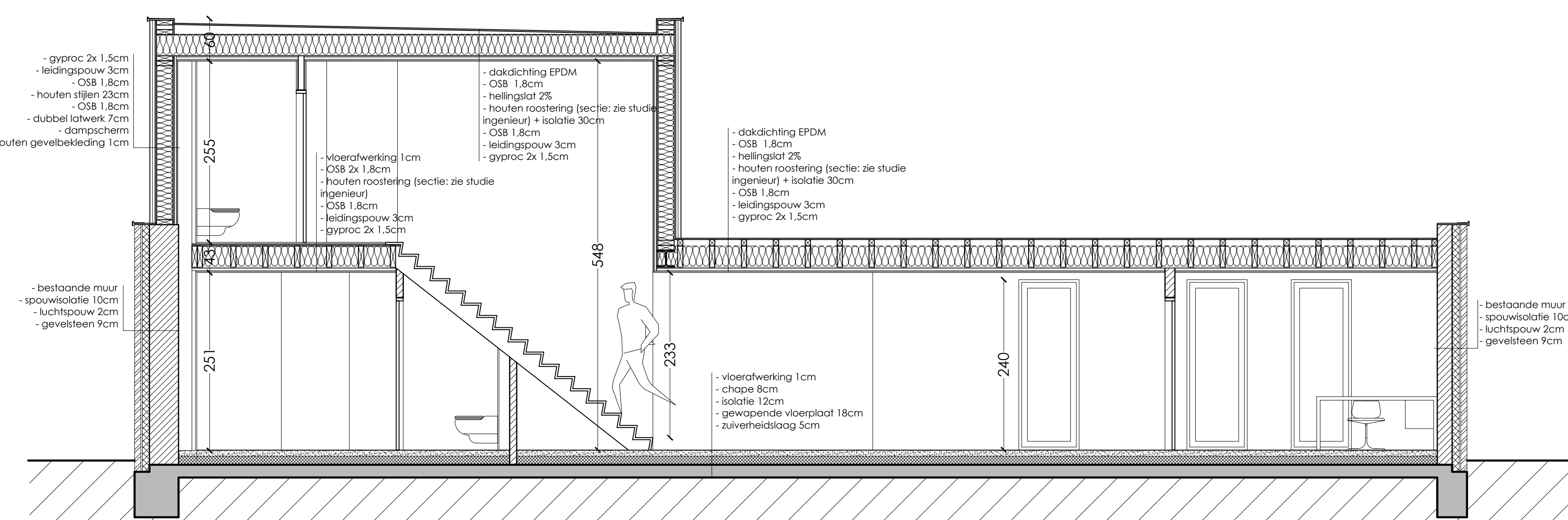
DOORSNEDE BB' _ 1/50
