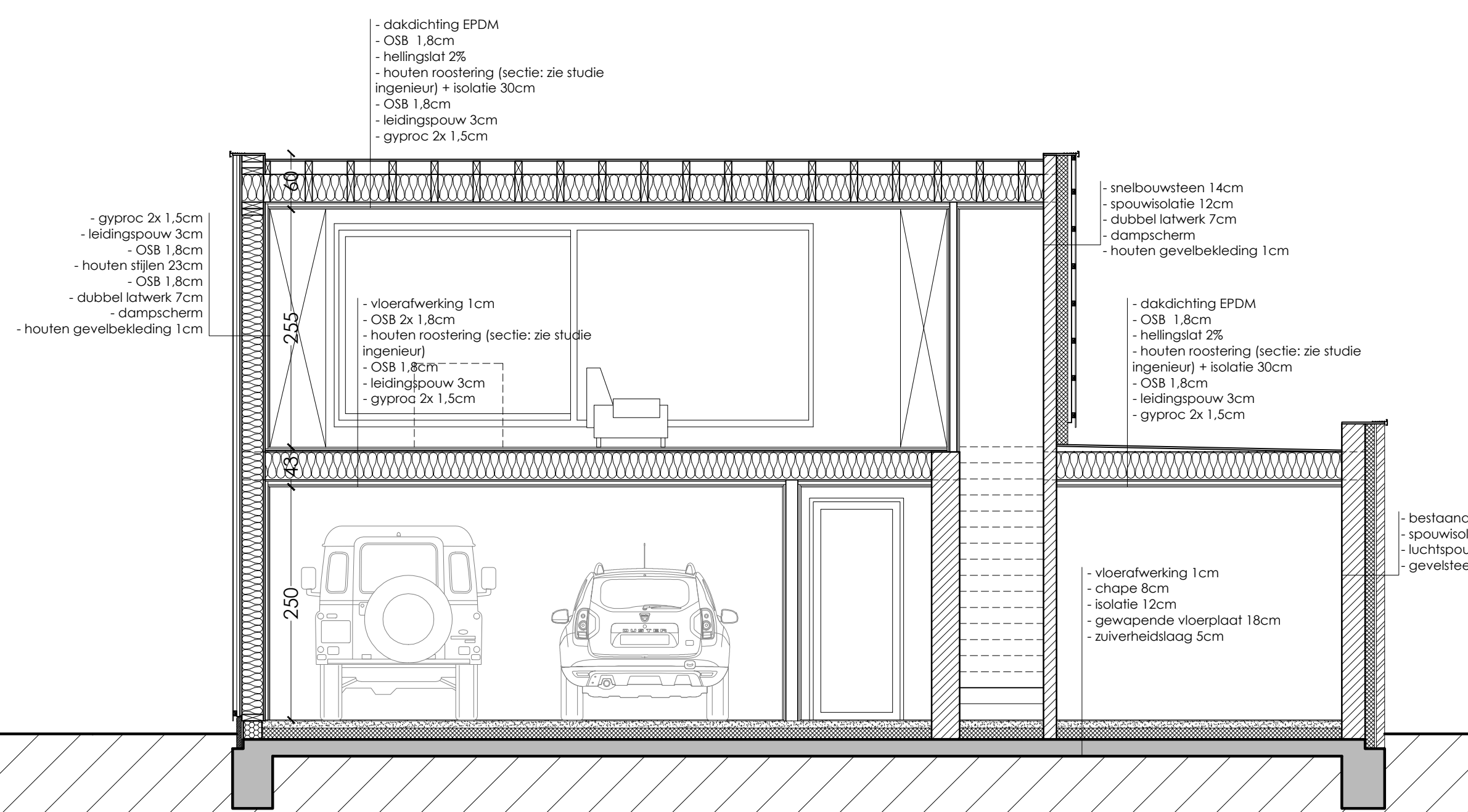
DOORSNEDE CC' _ 1/50
