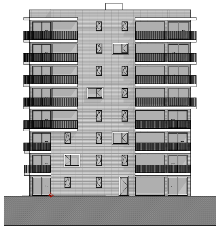
VOORGEVEL (PLEIN)
