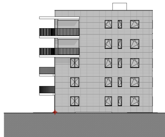
RECHTERGEVEL
