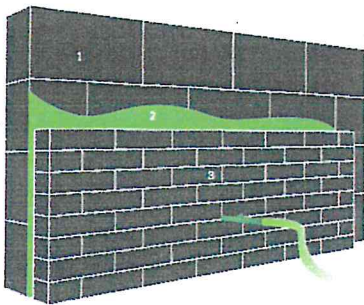
1. Dragende muur | 2. Ingeblazen isolatie | 3. Gevelsteen / gevelbekleding
