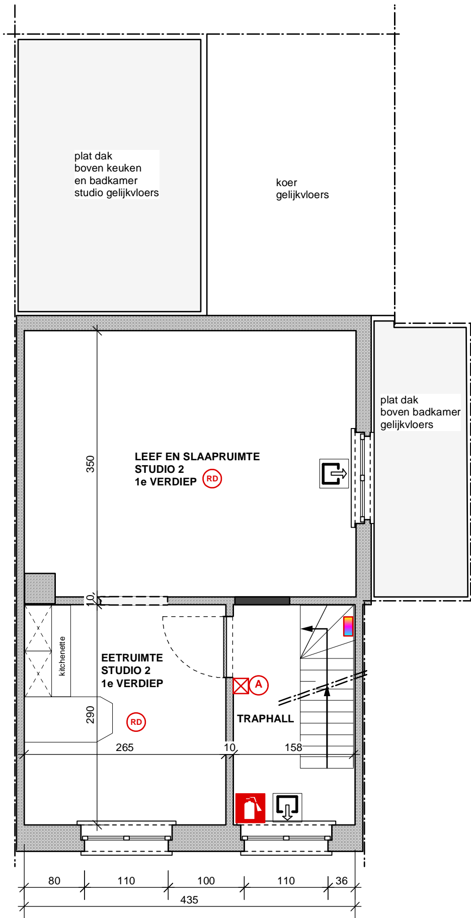
1e VERDIEPING - schaal 1/50 badkamer op het gelijkvloers
