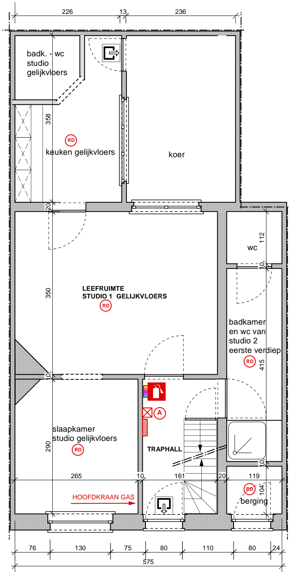
GELIJKVLOERS - schaal 1/50
