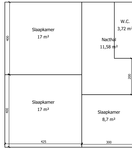
1ste verdieping
