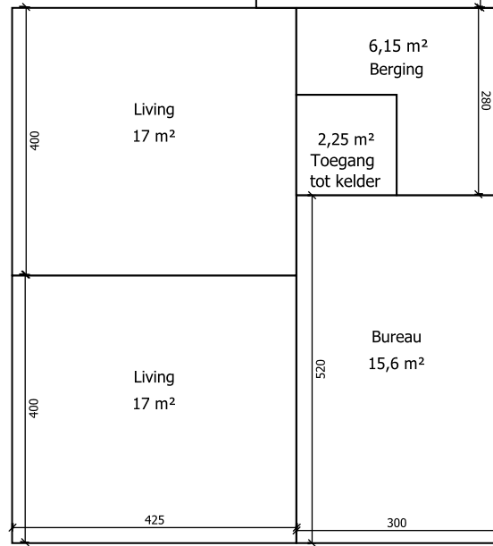
Gelijkvloers
