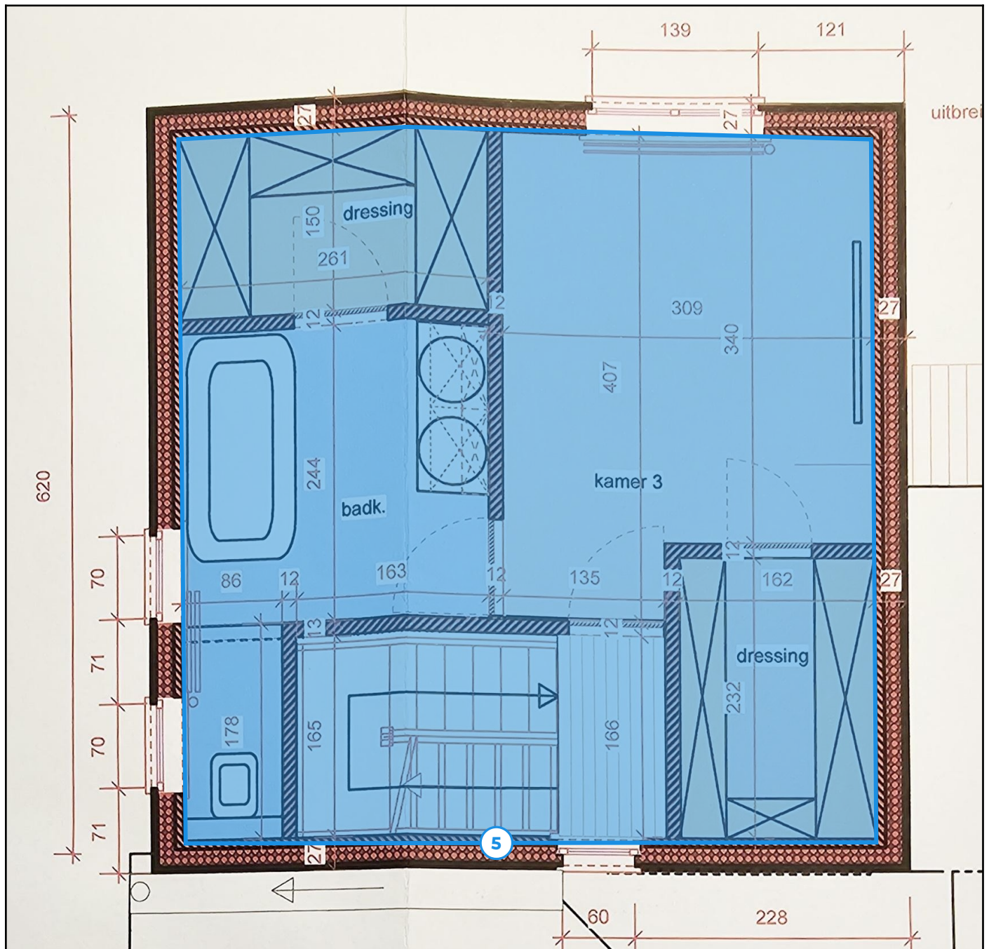
Legende van plan 1.4: Bovenverdieping plafond
