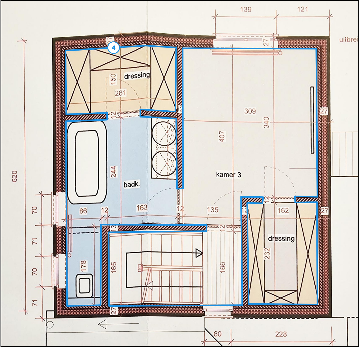
Legende van plan 1.2: Bovenverdieping
