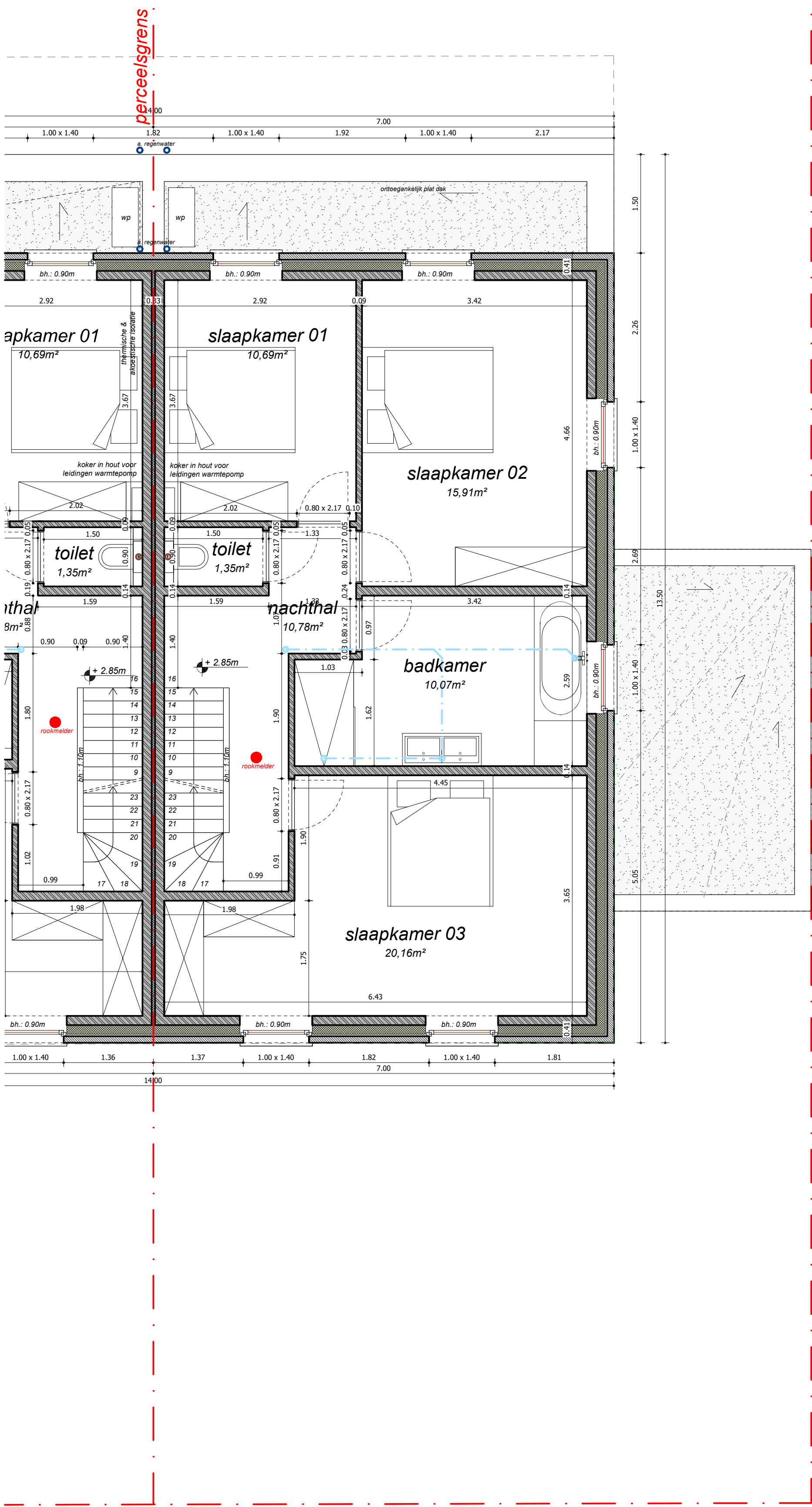
VERDIEPINGSPLAN
