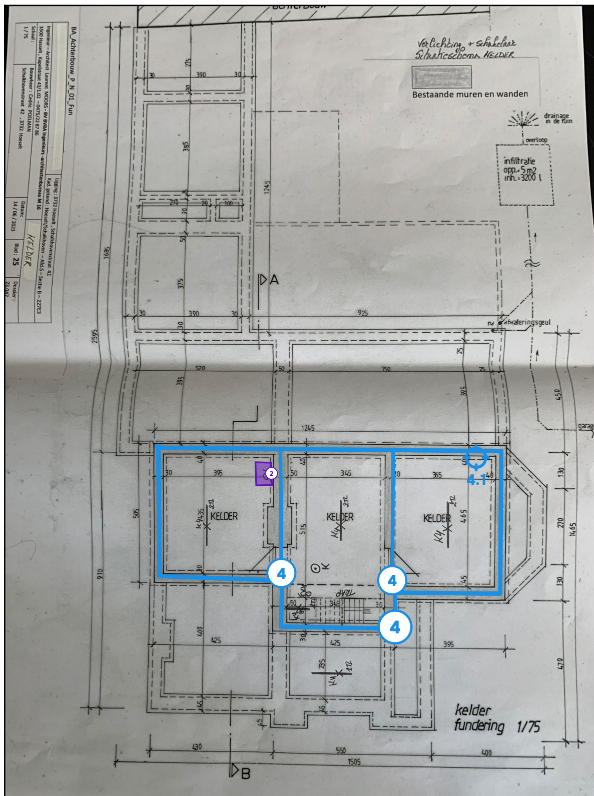
Legende van plan 1.1: Kelder; pleister wand en cv ketel
