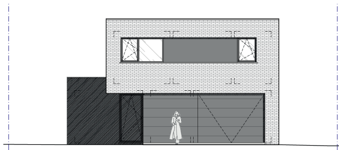
voorgevel
