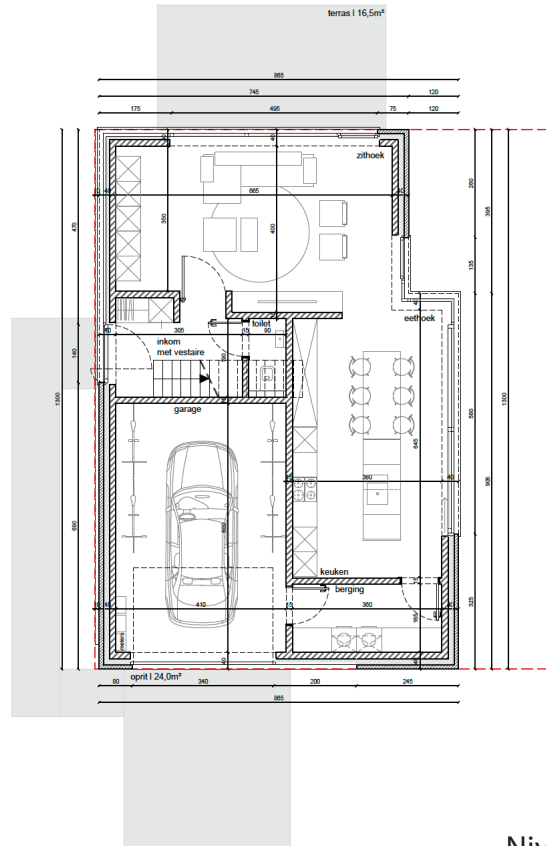
Nivo 0
