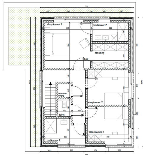
Nivo +1
