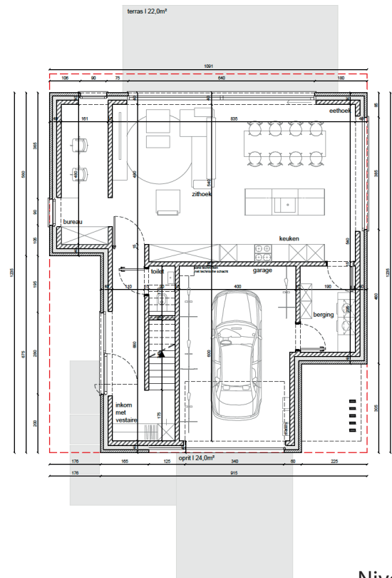
Nivo 0
