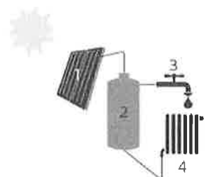
1. Zonnecollector | 2. Opslagvat zonneboiler | 3. Sanitair warm water | 4. Afgifte-element voor ruimteverwarming (radiatoren)
