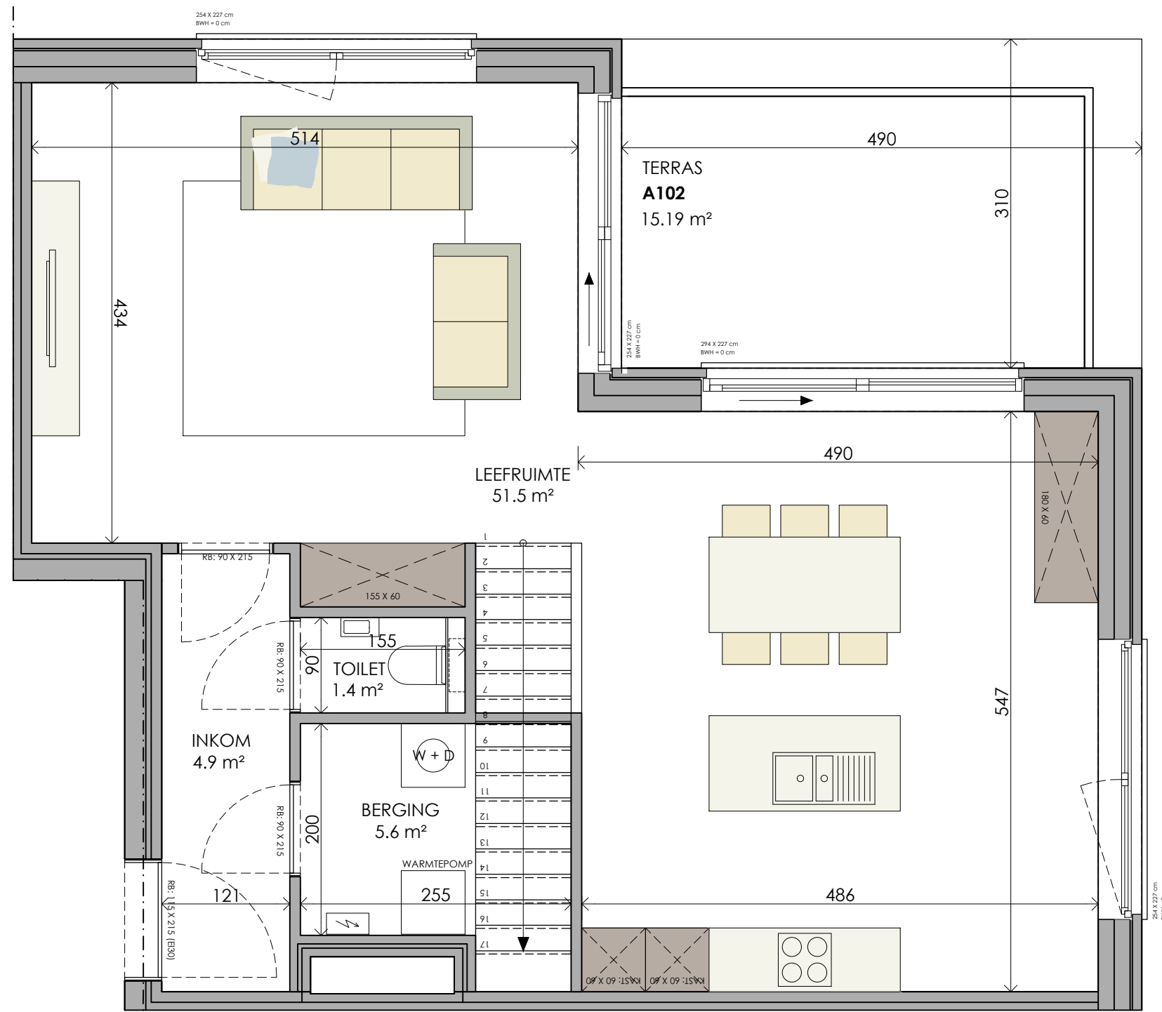
DUPLEX eerste verdieping
