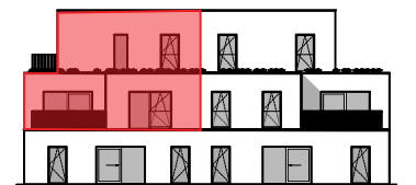
ACHTERGEVEL GEBOUW A
