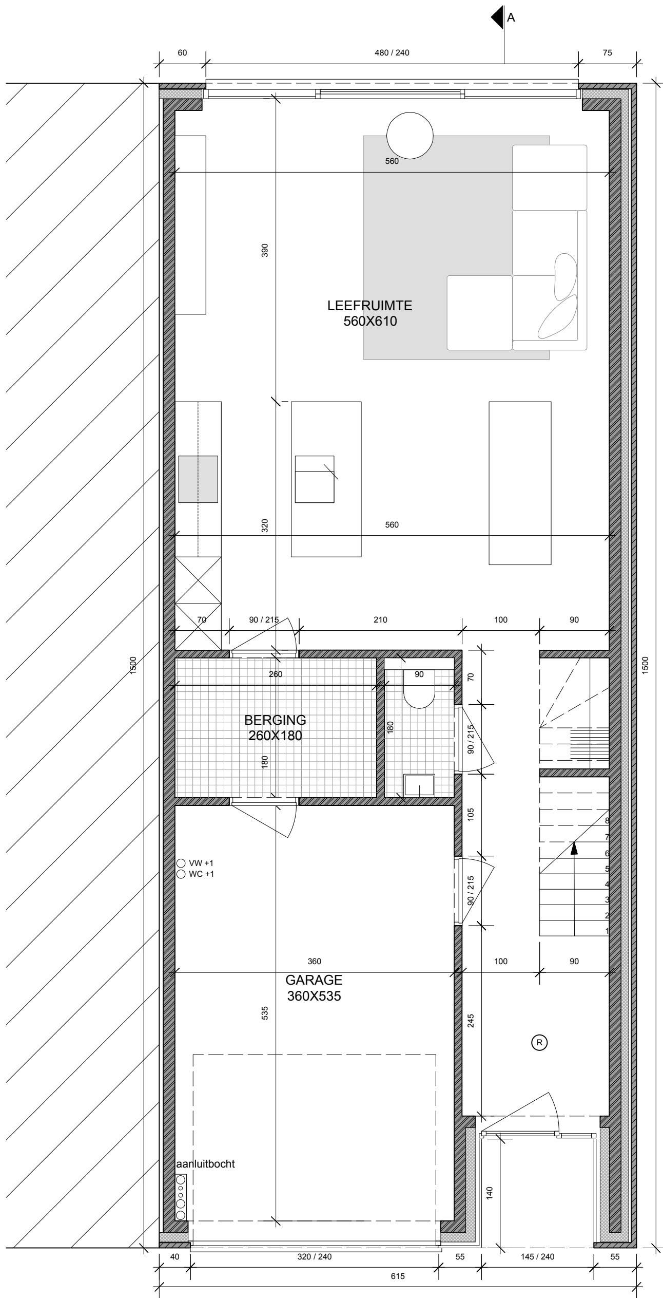
GRONDPLAN NIEUWE TOESTAND SCHAAL 1/50
