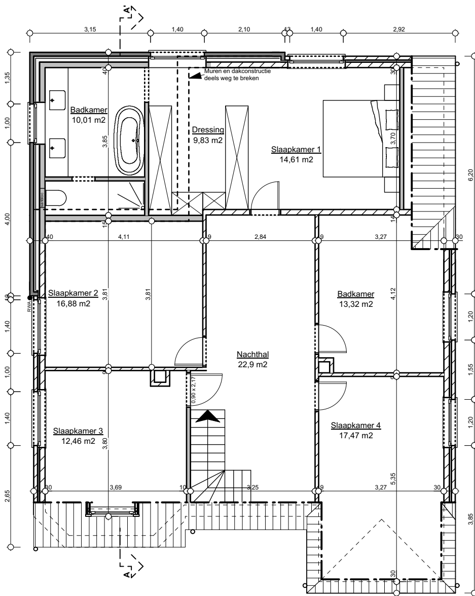
PLAN VERDIEPING Schaal 1/100
