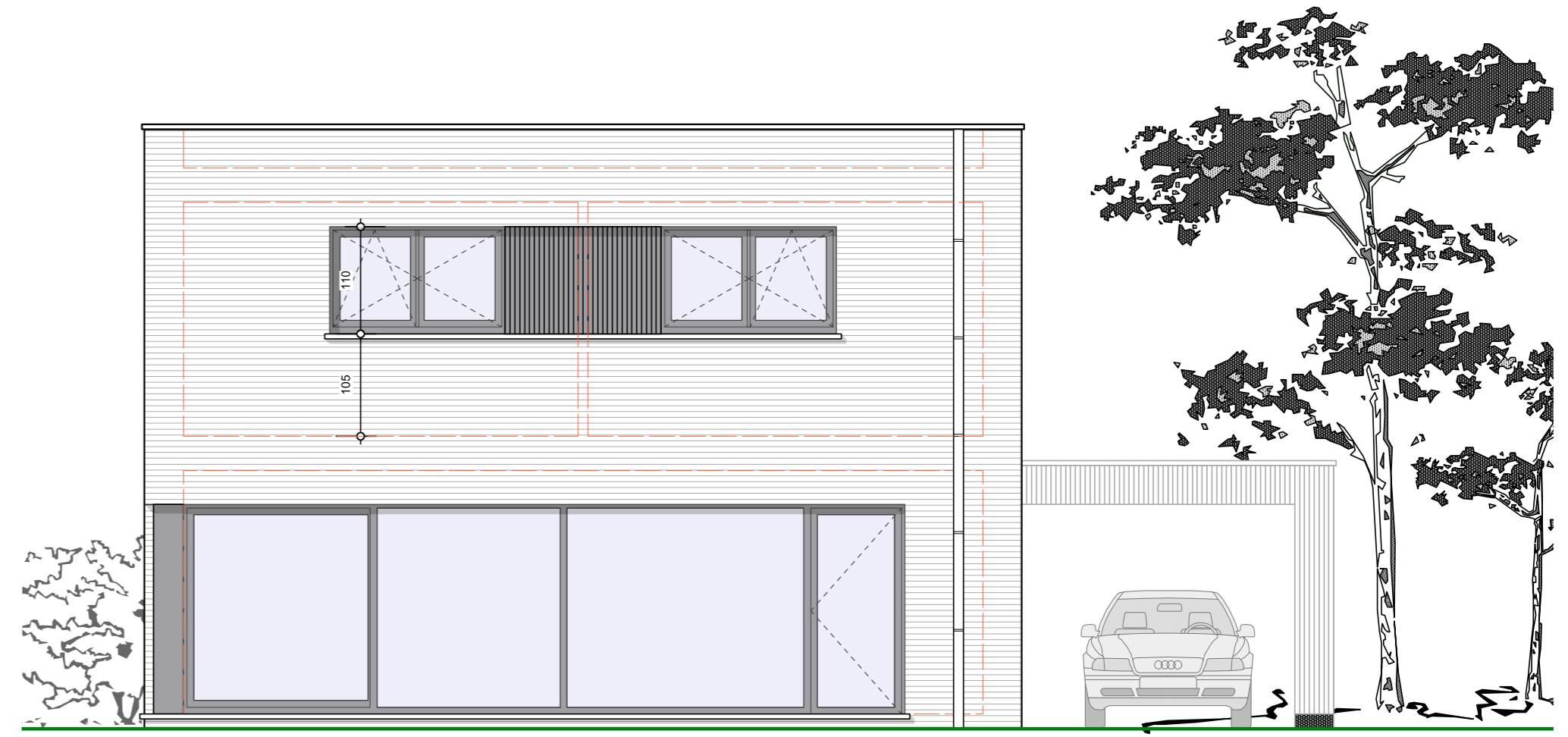
Achtergevel
