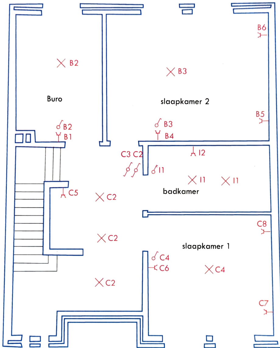
1 STE VERDIEPING
