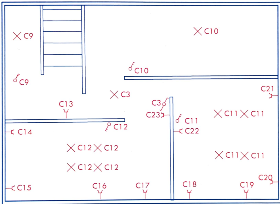
Zolderverdieping / STRAATZIJDE
