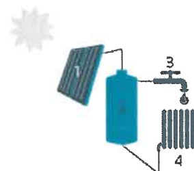
1 Zonnecollector | 2 Opslagvat zonneboiler | 3 Sanitair warm water | 4 Afsplittelement voor ruimteverwarming (optioneel)
