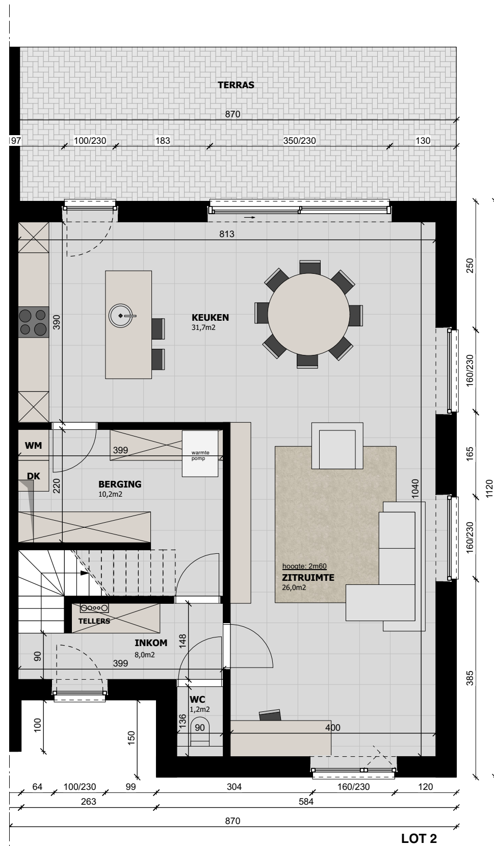
GELIJKVLOERS 1/75
