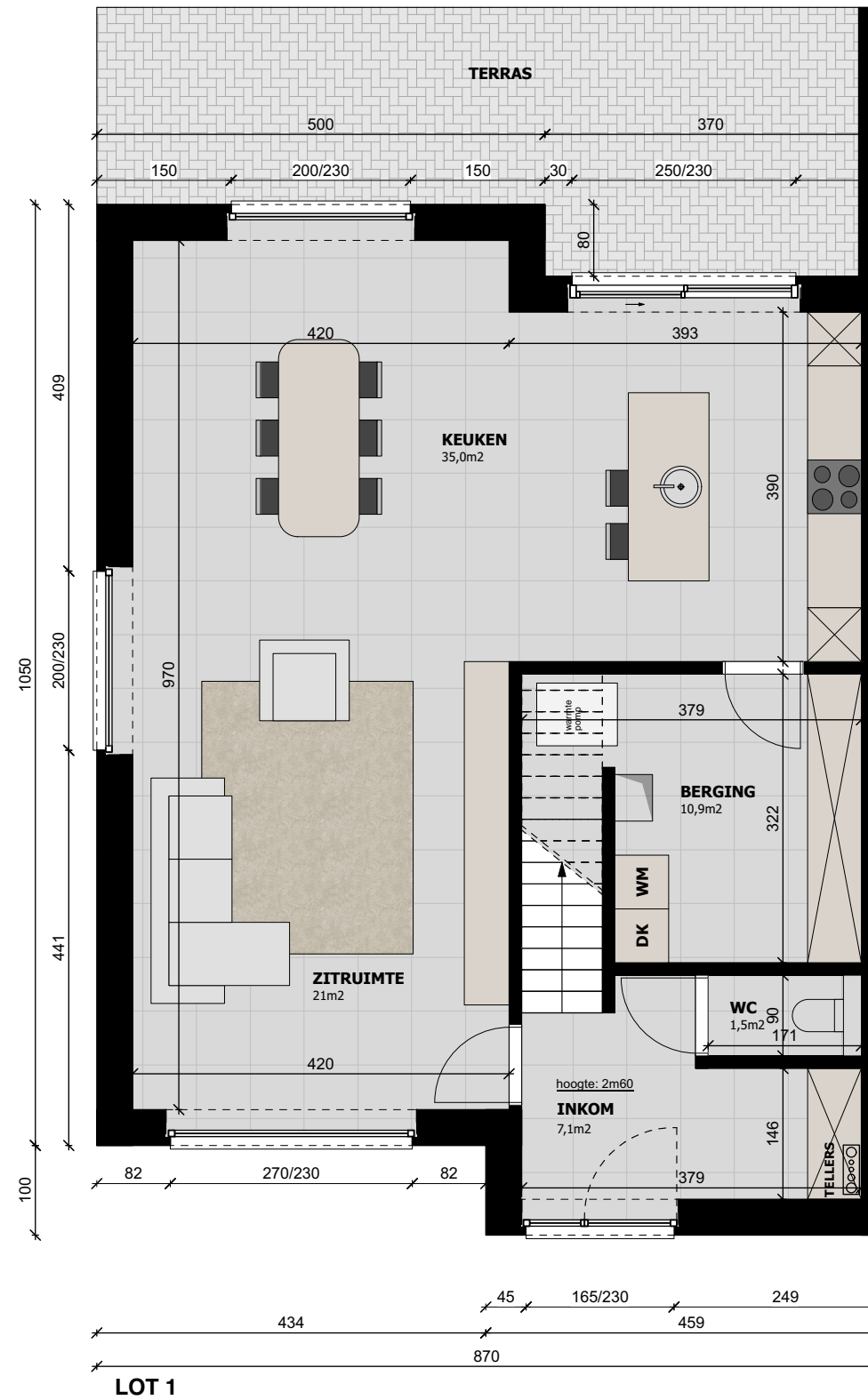
GELIJKVLOERS 1/75
