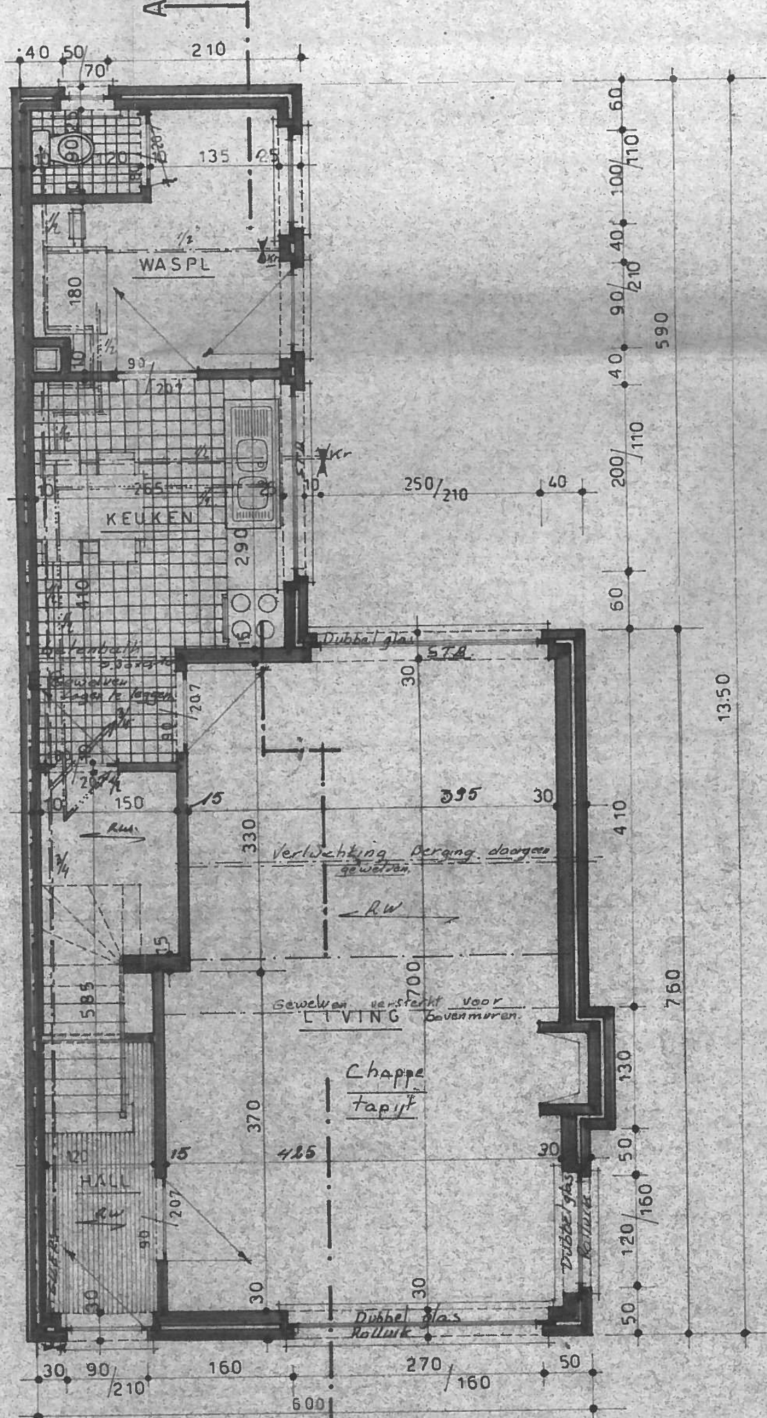
GRONDPLAN
