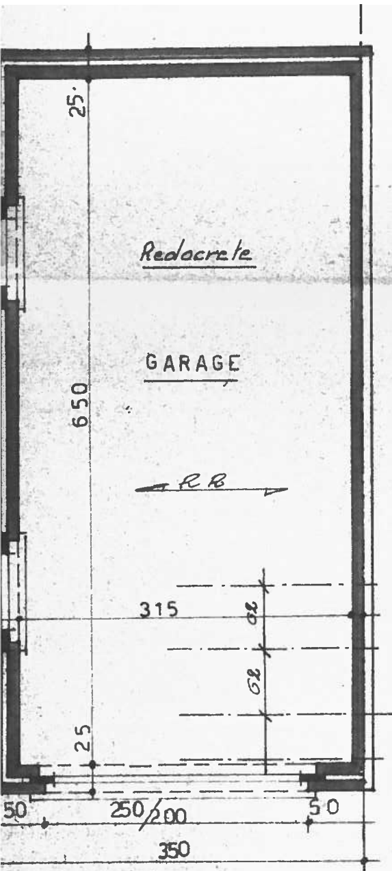
GRONDPLAN
