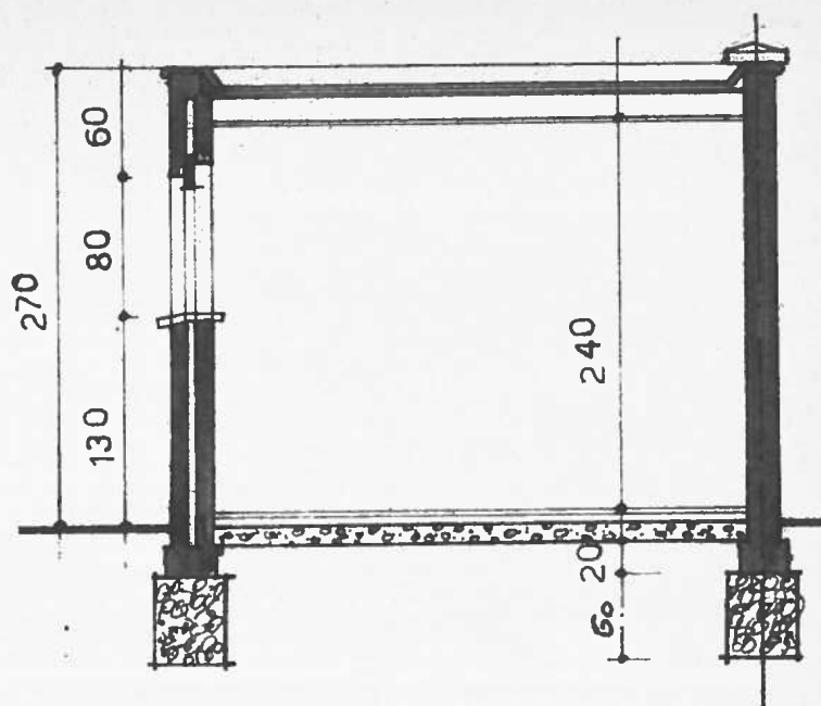
DOORSNEDE
