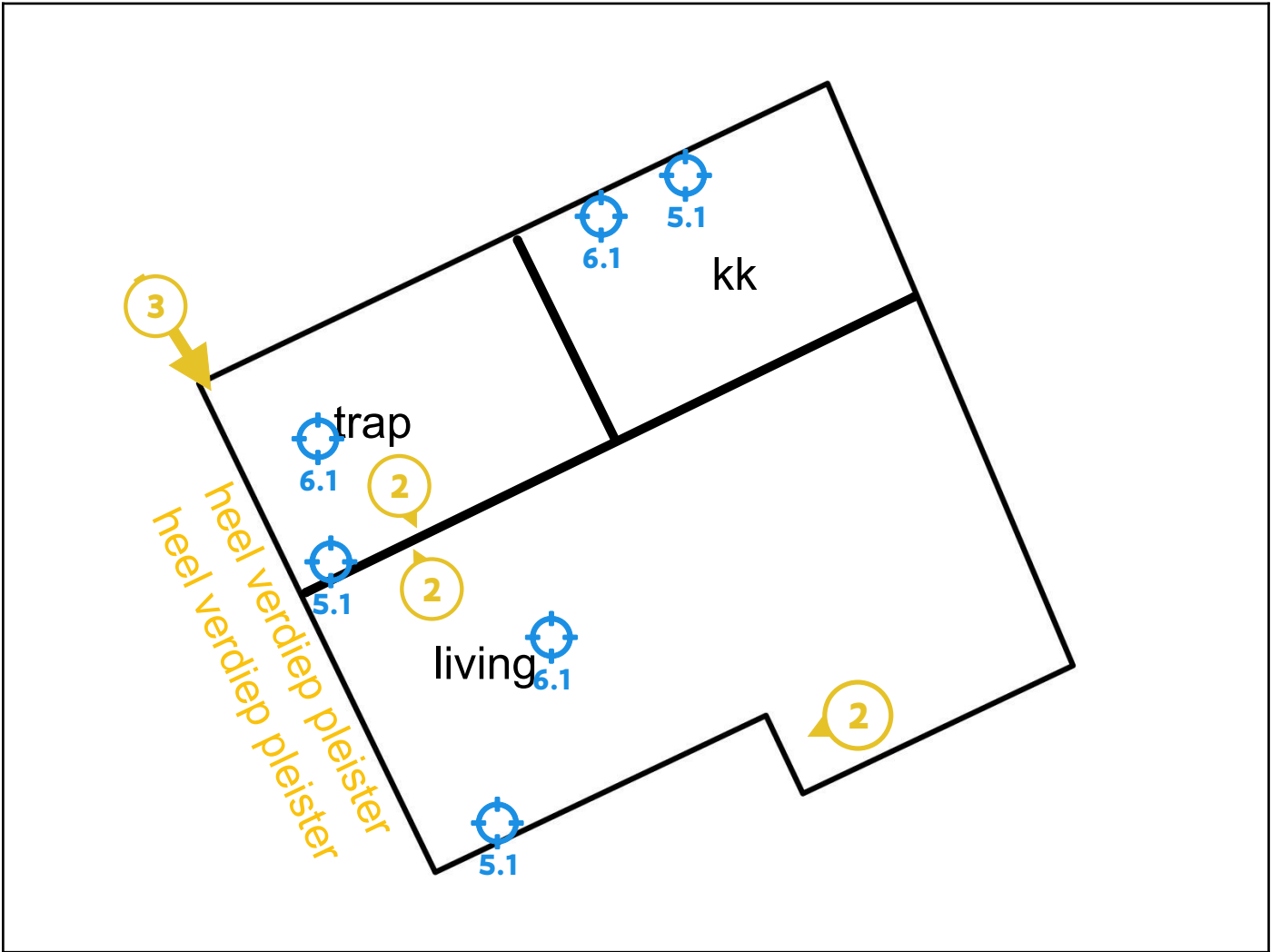
Legende van plan 1.1: Hoofdgebouw plan gvl
